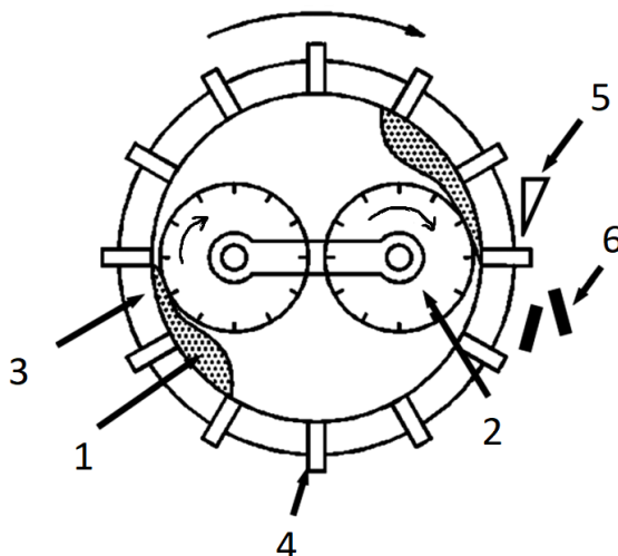
Obr. 9 - Granulátor
