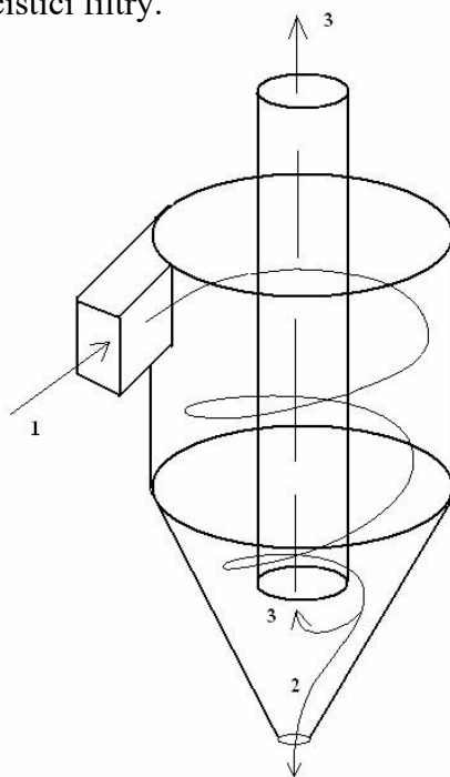
Obr. 5 - Schéma cyklonu
