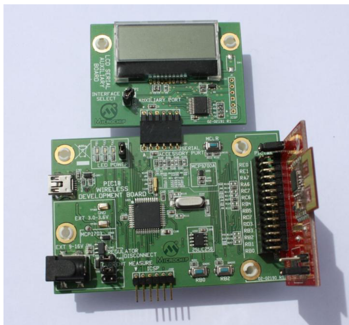
Obr. 8: Vývojová deska použitá pro implementaci akčního členu Kotel.
