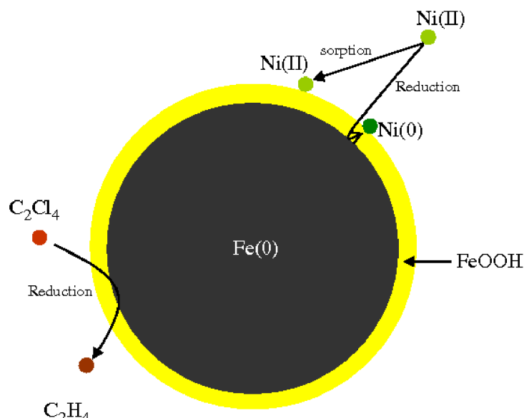
Obr. 2: Core-shell struktura nZVI částice ve vodném prostředí. [25]
