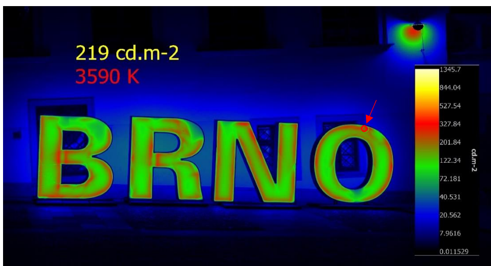
Obrázek 6.16 Světelná reklama 40-1B
