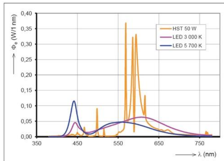
Obrázek 3.2 Rozložení energie pro různé zdroje záření [23]
