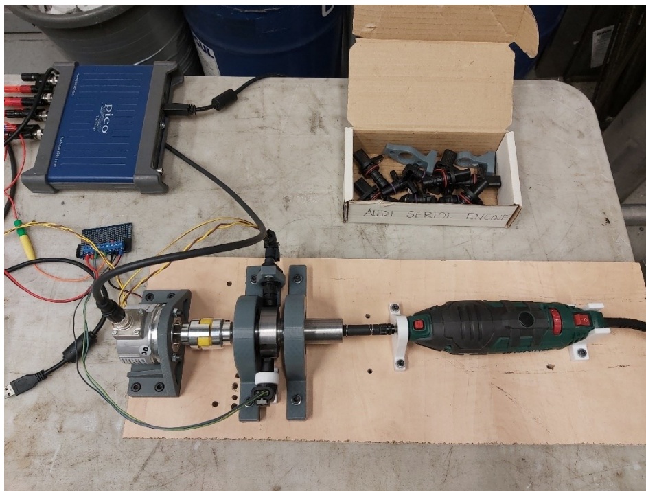
Obrázok 37 Meracia aparatura
