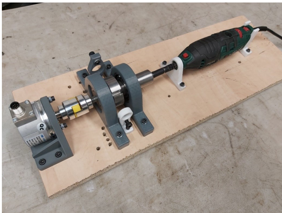
Obrázok 25 Meracie zariadenie
