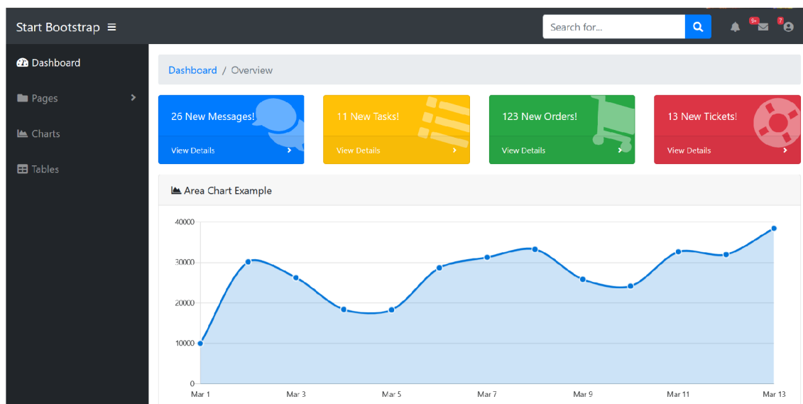
Obr. 2.4: Vzor GUI
