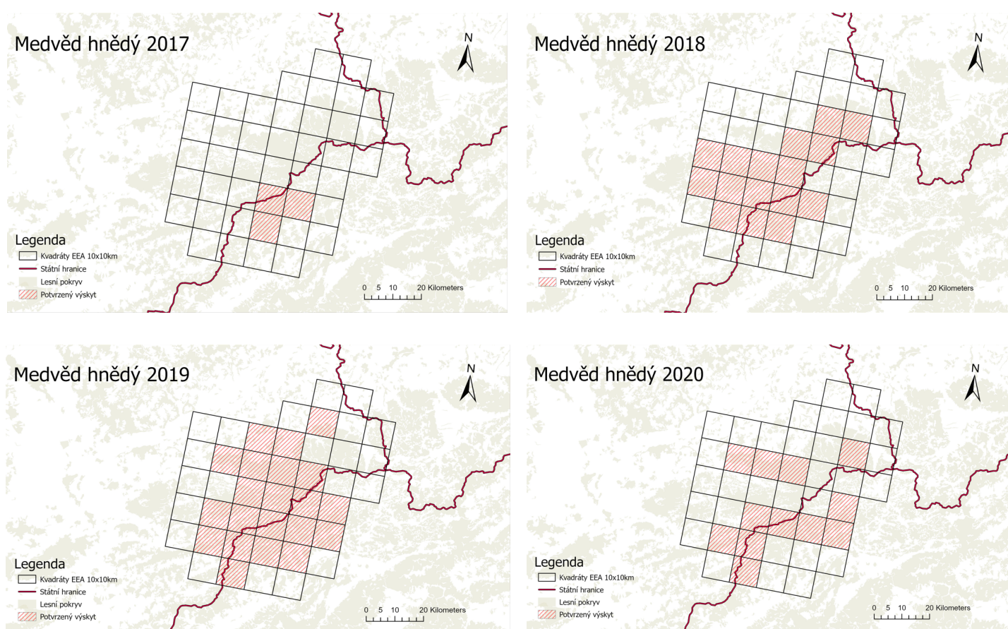
Obr. 12: Mapy výskytu medvěda hnědého na československém pomezí v letech 2017–2020. Každá mapa představuje jeden kalendářní rok.
