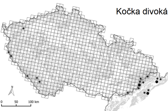
Obr. 3: Srovnání map výskytu medvěda hnědého, rysa ostrovida a kočky divoké na našem území dle Nálezové databáze ochrany přírody (AOPK 2022) a Kutala et al. (2017). Nalevo jsou mapové výstupy z Nálezové databáze ochrany přírody, napravo z Kutal et al. (2017).
