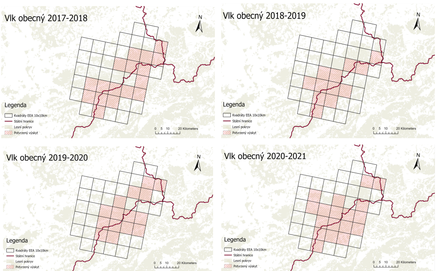
Obr.13: Mapy výskytu vlka obecného na československém pomezí v letech 2017–2021. Každá mapa představuje jeden rysí rok, který začíná 1.5. daného roku a končí 30.4. následující roku.
