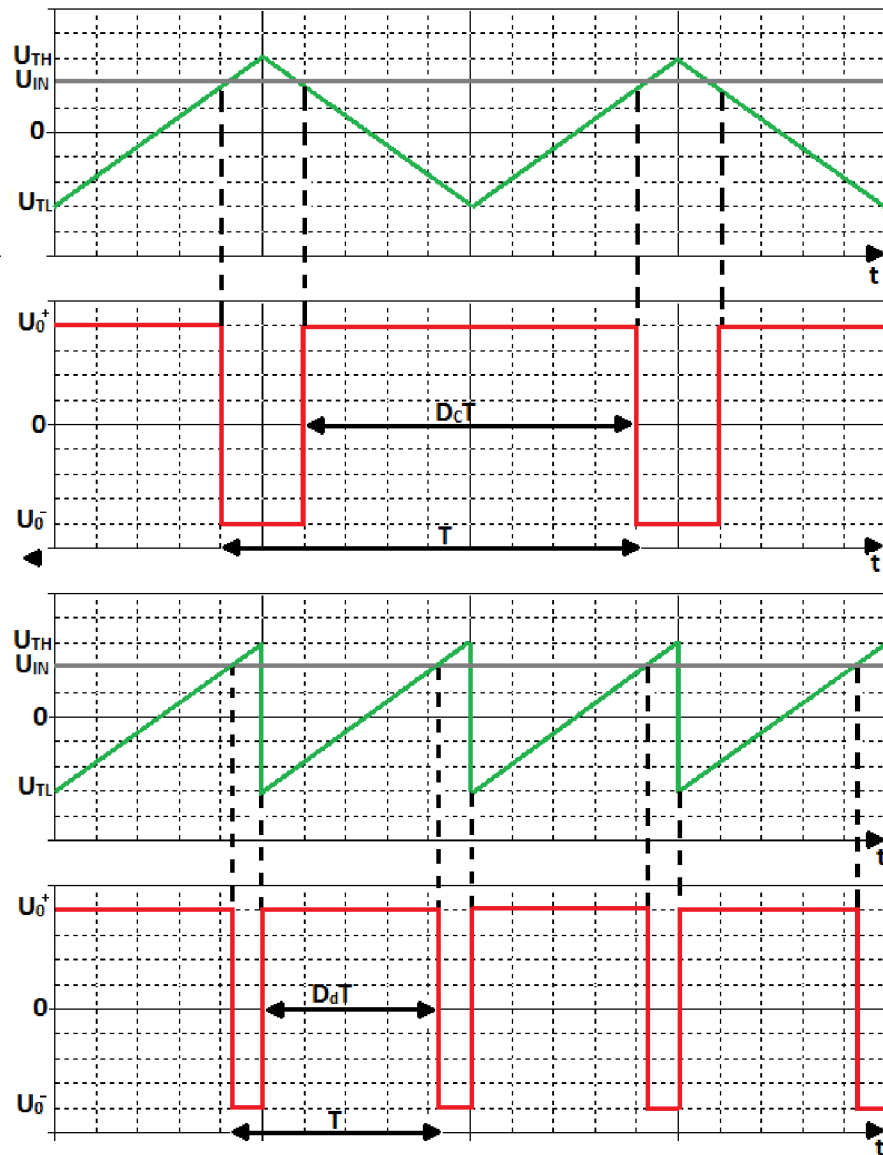
Obrázek 2.8 Časové průběhy modulace modulátoru s DVCC
