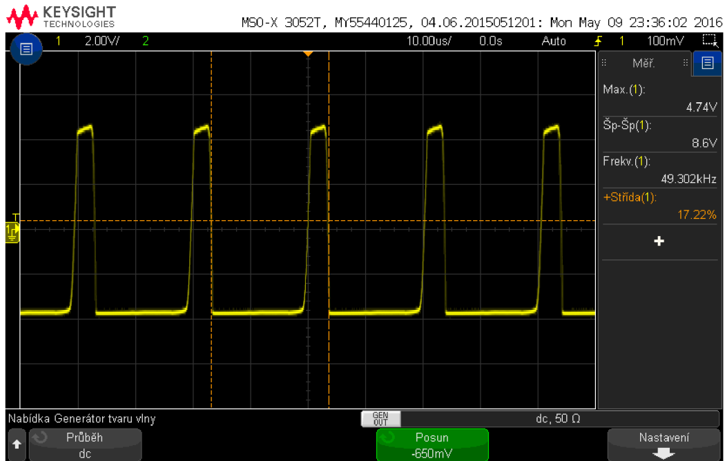
Obrázek 4.12 Minimální střída modulátoru (změřeného)
