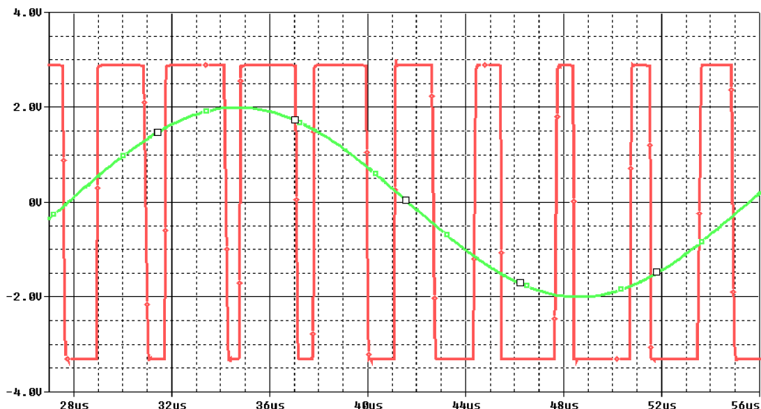
Obrázek 4.19 Simulovaná PWM modulace
