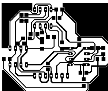
Obrazec plošného spoje ze strany mědic 1:1
