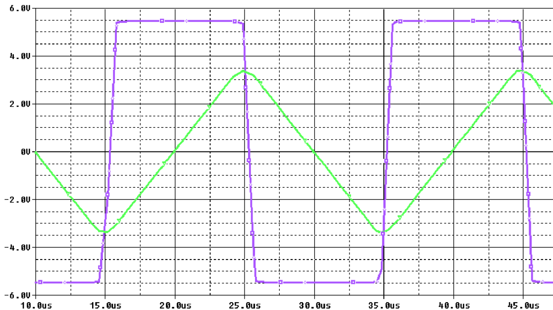
Obrázek 3.4 Obdelníkový a trojúhelníkový průběh modulátoru řízeného konvejorem
