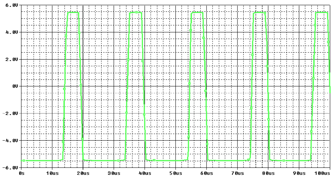
Obrázek 4.13 Minimální střída modulátoru (simulovaného)
