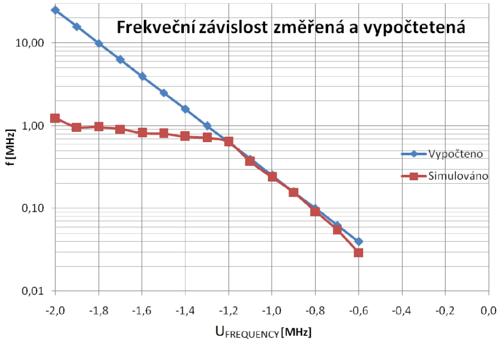
Obrázek 4.18 Frekvenční průběh modulátoru s diamantovým tranzistorem
