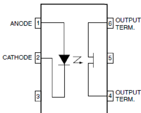
Obrázek 2.6 H11F1 v pouzdře DIP8 převzato z [10]
