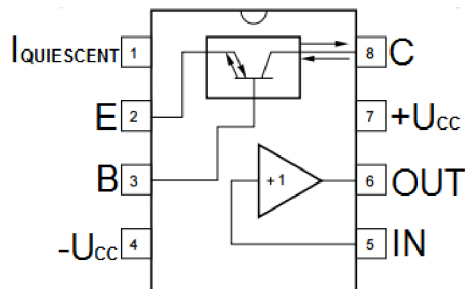
Obrázek 2.3 Rozvrhnutí OPA660 v pouzdře DIP8 (horní část diamantový tranzistor), převzato z [5]
