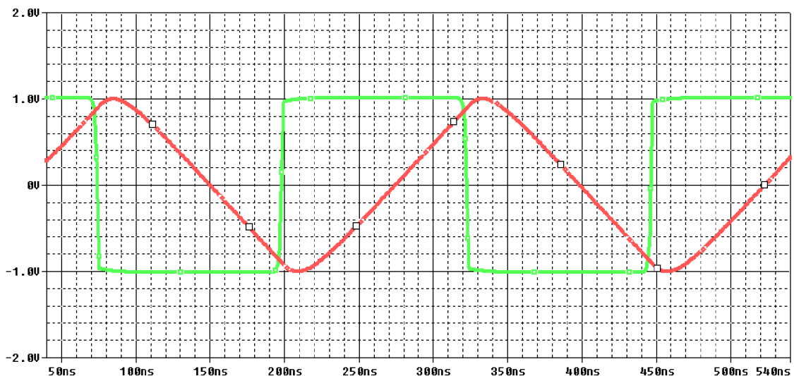
Obrázek 4.1 Obdélníkový a trojúhelníkový průběh výstupů modulátoru simulovaný
