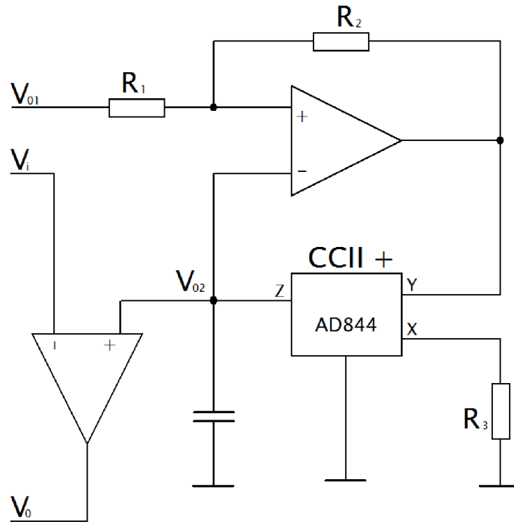
Obrázek 2.9 Schéma zapojení PWM Siripruchyanunova modulátoru
