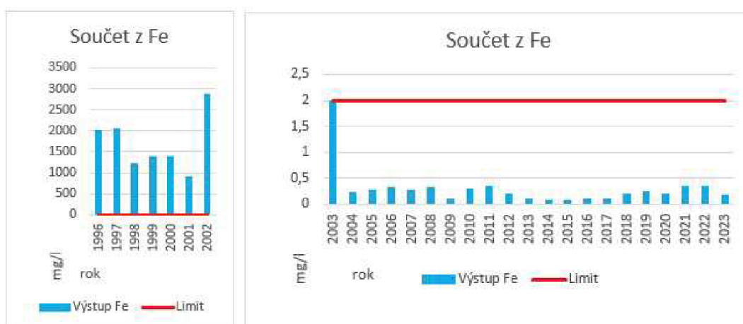
Obr. 46: Výstupní hodnota Fe do ČDV (1996 – 2023)
