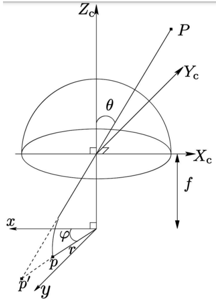
Obrázek 3.2: Rozdíl modelu perspektivní projekce od modelu kamery typu rybího oka Převzato z [1]
