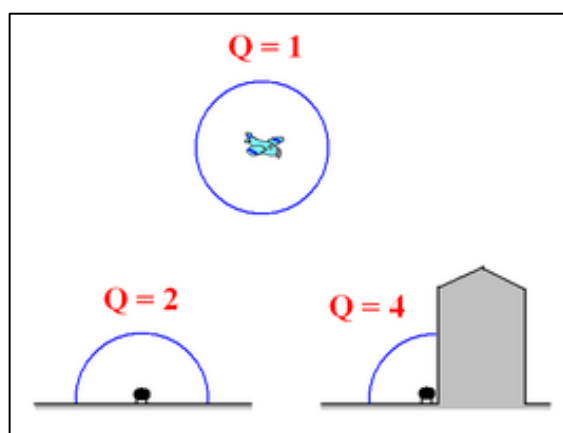
Obrázek 11 – typické hodnoty činitele Q [-] (12)
