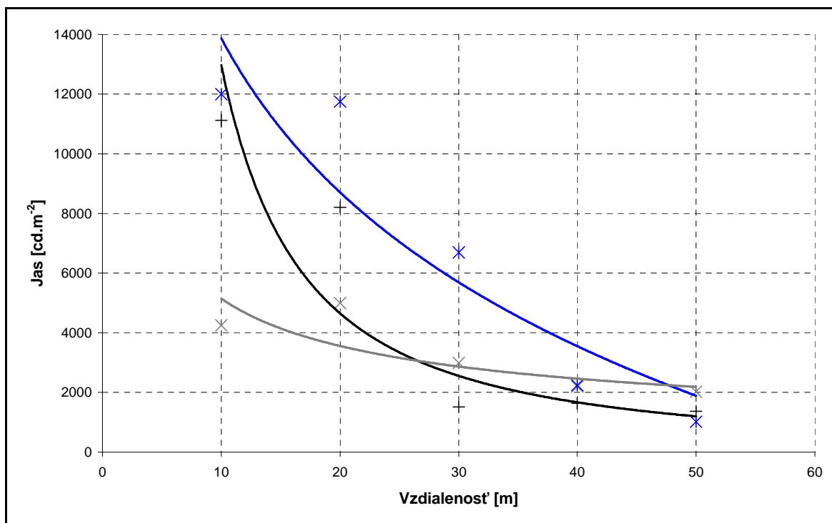
Obr. č. 4 – 31 porovnanie jasov kombinácie obrysových, brzdoých a smerových svetiel jednotlivých vozidiel
