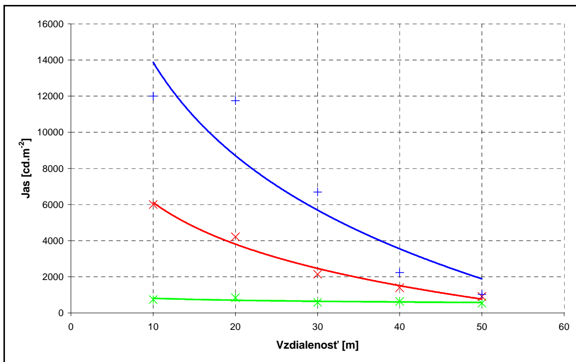
Obr. č. 4 – 27 Závislosť jasů svetiel na vzdialenosťi pre vozidlo Škoda Octavia II
