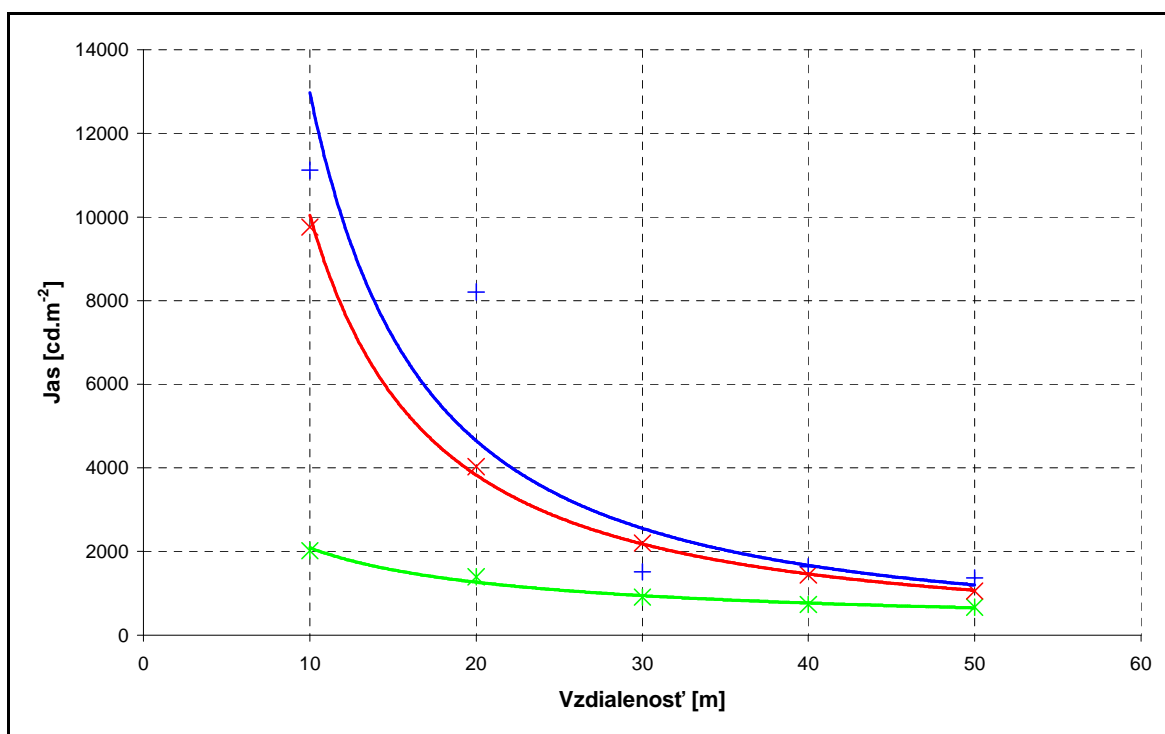
Obr. č. 4 – 28 Závislosť jasů svetiel na vzdialenosťi pre vozidlo Volkswagen Sharan
