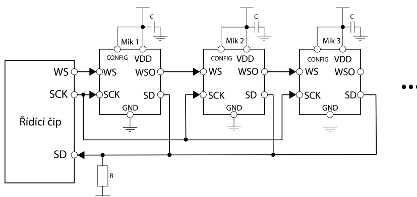
Obr. 3.2: Zapojení mikrofónů ICS-52000 [33].
