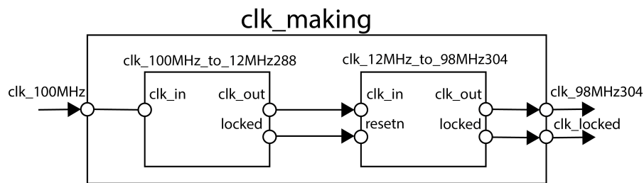
Obr. 4.2: Zapojení clk_making .
