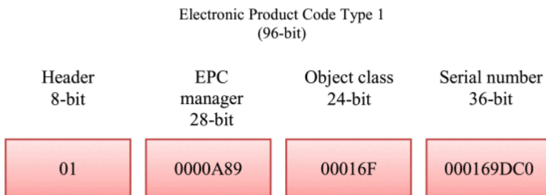
obrázek č. 22 – Ukázka EPC [22]
