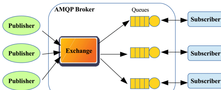
obrázek č. 12 – Architektura protokolu AMQP [12]
