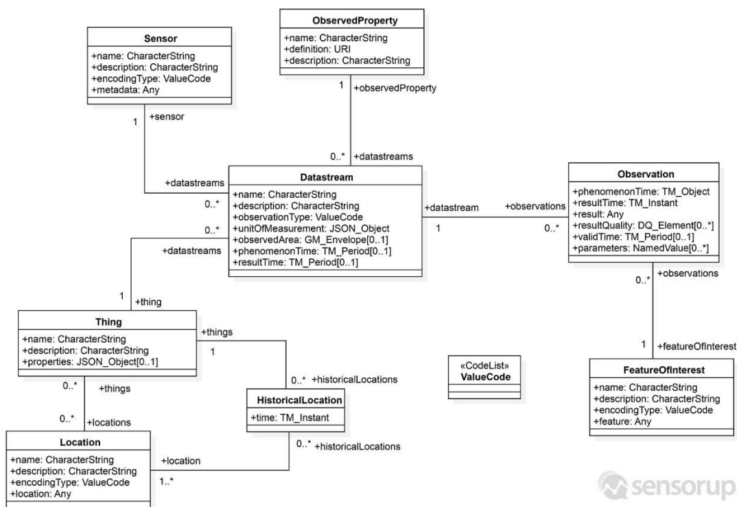
obrázek č. 36 – SensorThings API UML diagram [36]
