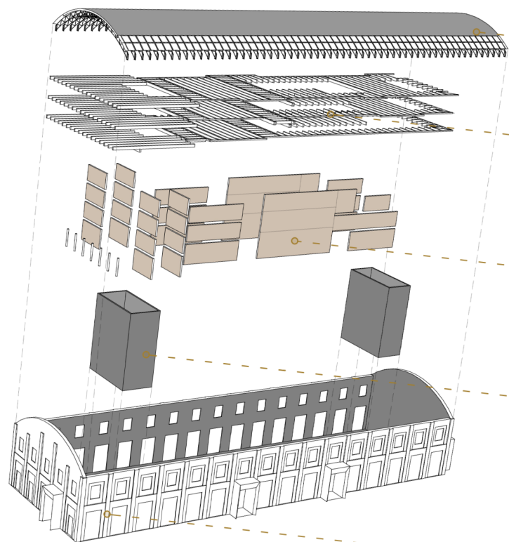
Schéma konstrukce
