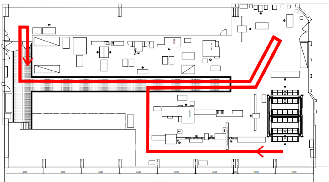
Obr. 11 Grafické znázornění pohybu představitele 2 po dílně.
