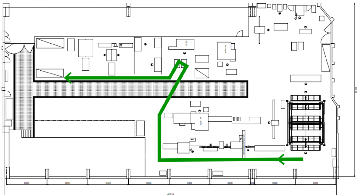
Obr. 33 Grafické znázornění pohybu představitel 2 v navrženém dispozičním řešení.
