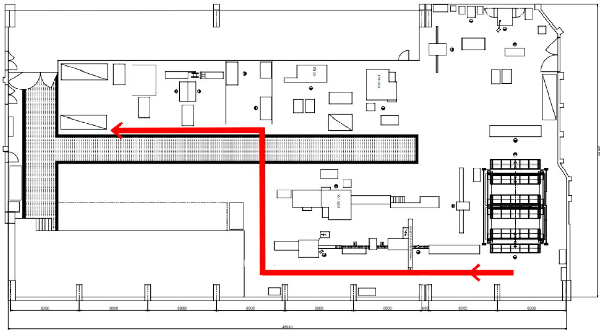
Obr. 32 Grafické znázornění pohybu představitel 1 v navrženém dispozičním řešení.
