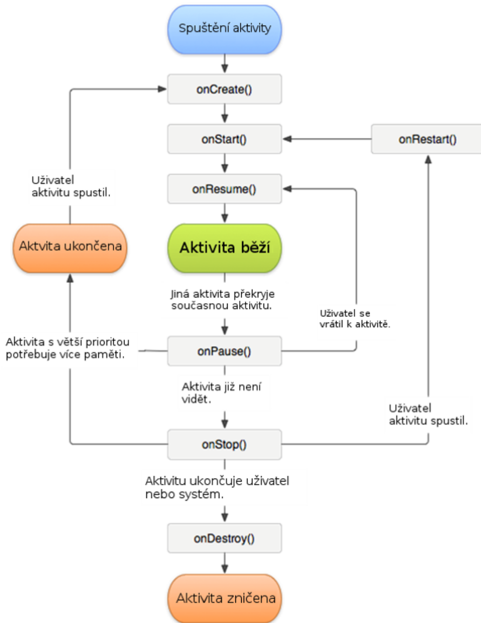
Obrázek 8: Schéma životního cyklu
