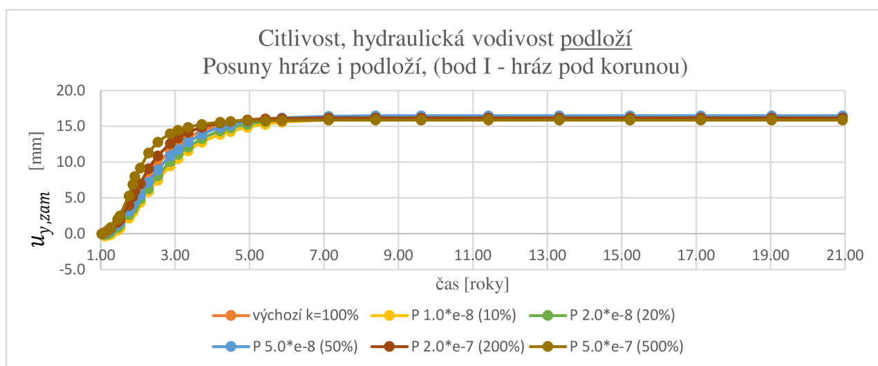
Obrázek 7.11 Porovnání citlivosti celkových vertikálních posunů u_{y,zam} na hydraulickou vodivost podloží v jednotlivých částech.
