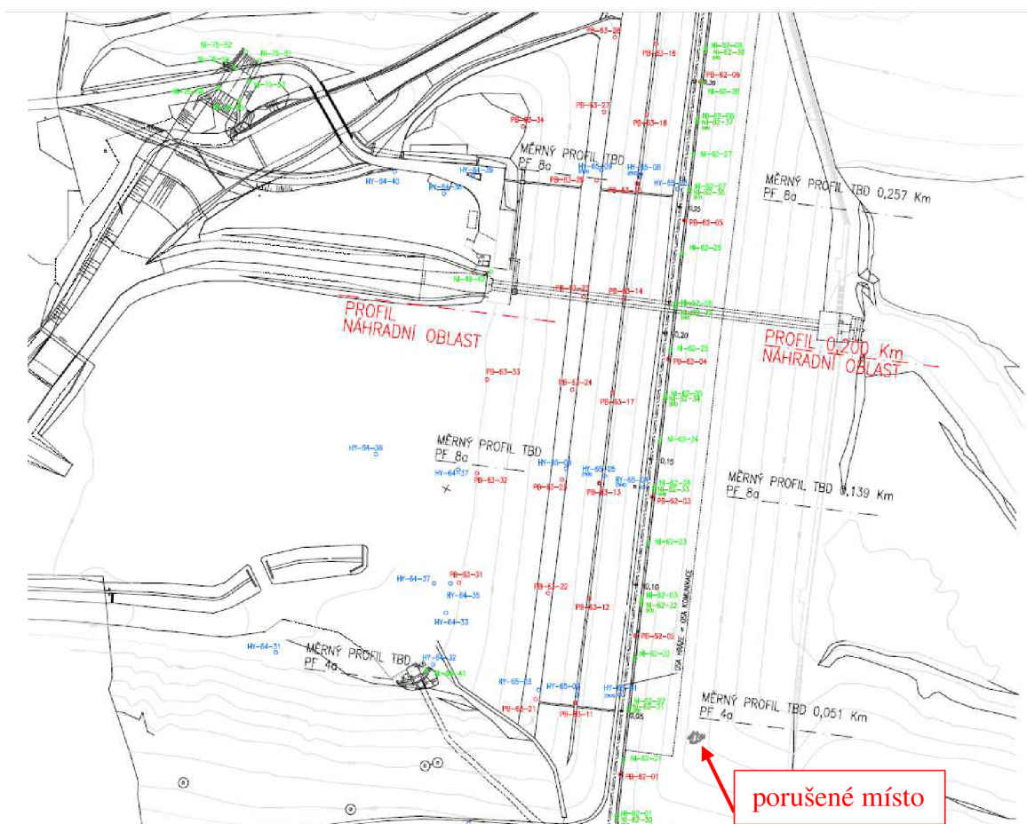
Obrázek 8.5 Schéma situace hráze VD Morávka [Rainer, 2012]
