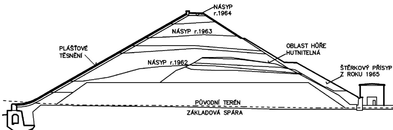
Obrázek 8.1 Rozdělení tělesa hráze na sypací vrstvy
