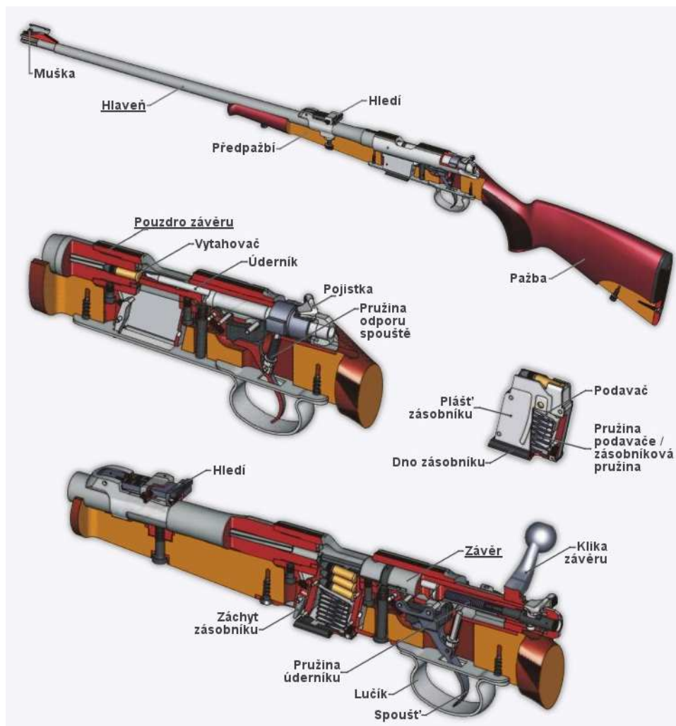
Obrázek 2: Malorážka ZKM 451
