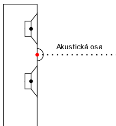
Obr. 1.8: Zobrazení akustické osy soustavy s uspořádáním D'Appolito, tato osa je pro všechny kmitočty shodná
