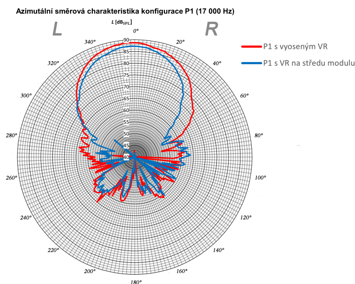
Obr. 5.5: Azimutální směrová charakteristika konfigurace P1 s VR na středu modulu a vyoseným VR (pohled shora), měřeno na kmitočtu 17 000 Hz
