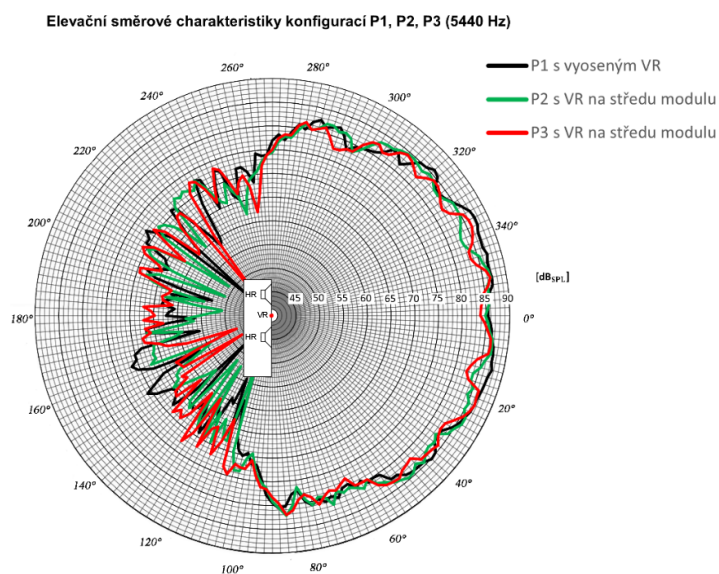
Obr. 5.8: Elevační směrová charakteristika konfigurací P1 s vyoseným VR a P2 a P3 s VR na středu modulu (s naznačením orientace reproduktorové soustavy), měřeno na kmitočtu 5440 Hz
