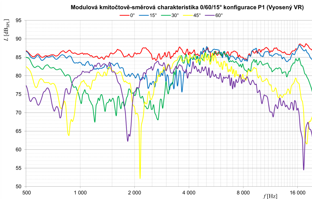
Obr. 5.9: Elevační kmitočtově-směrová charakteristika konfigurace P1 s vyoseným VR, měřeno mezi úhly 0° a 60° (kroku 15°)
