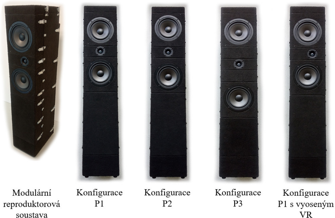
Obr. 3.1: Modulární reproduktorová soustava s různými konfiguracemi modulů
