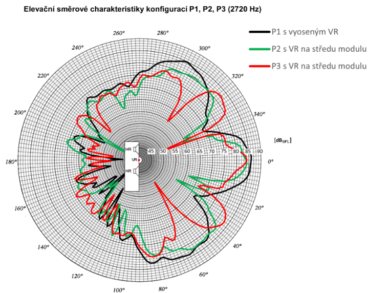
Obr. 5.7: Elevační směrová charakteristika konfigurací P1 s vyoseným VR a P2 a P3 s VR na středu modulu (s naznačením orientace reproduktorové soustavy), měřeno na mezním kmitočtu 2720 Hz
