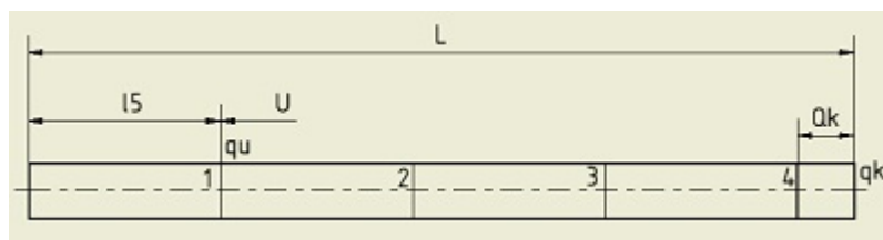
Obr. 4.1 Ztráty materiálu dělením tyčí a obráběním [1, 7].
