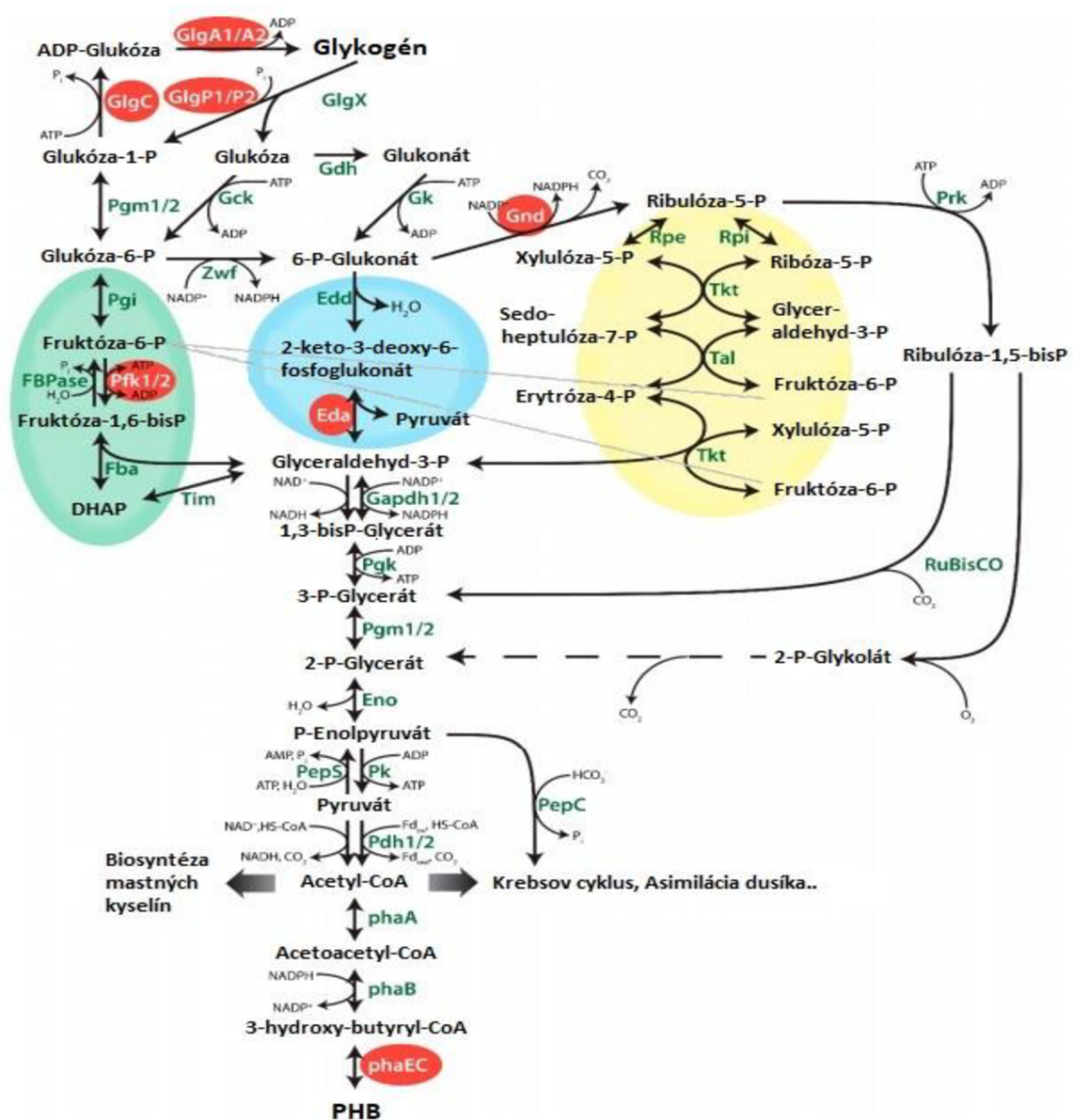
Obrázok 8 - Grafické vyobrazenie metabolizmu prekursorov PHB u Synechocystis , s červeným označením mutovaných/deletovaných génov rámci experimentov a vyobrazením EMP zelenou, ED modrou a OPP žltou farbou. Prevzaté, upravené z [138].
