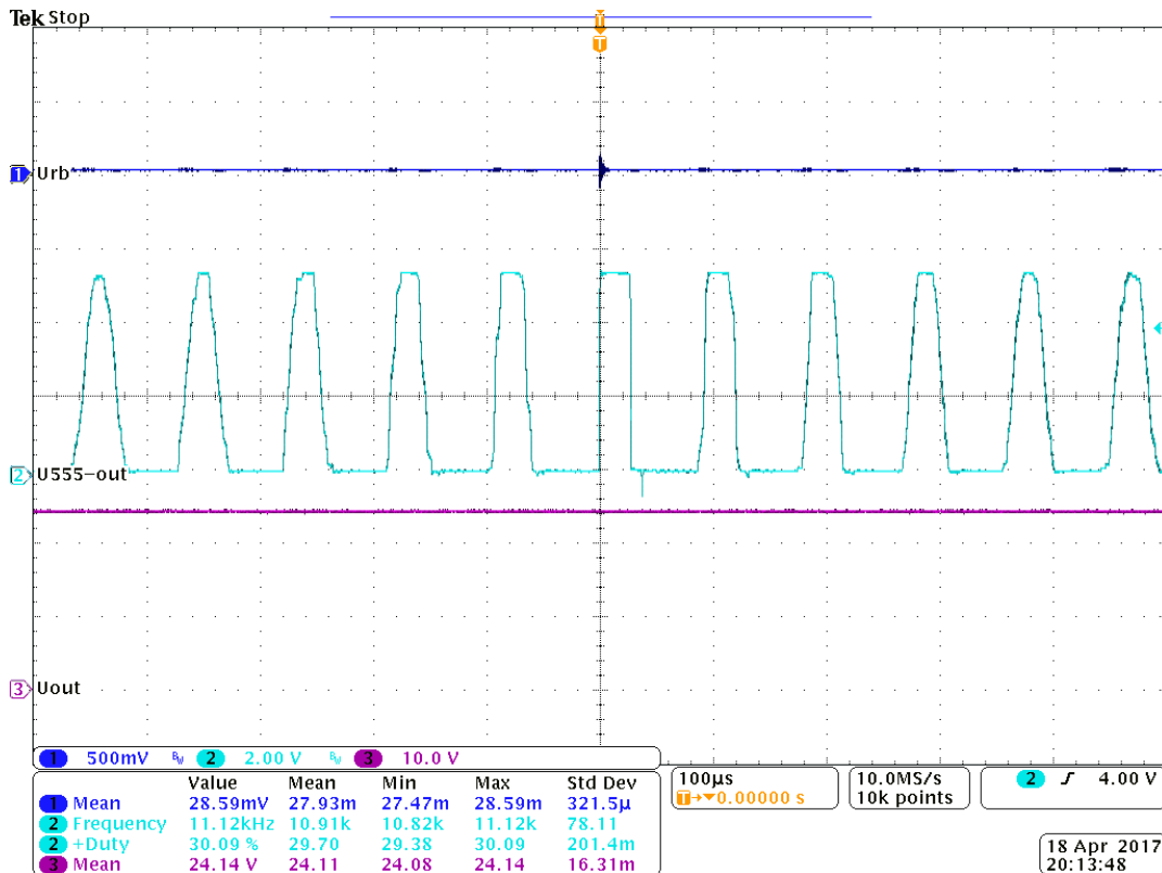
Obr. 25: Časové průběhy proudu (modře) spínacího signálu (zeleně) a výstupního napětí (fialově) zvyšujícího zatíženého měniče s obvodem 555 – zátěž 15 kΩ
