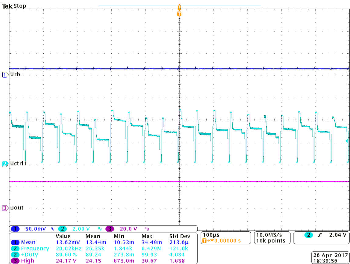
Obr. 39: Časové průběhy proudu (modře), spínacího signálu (zeleně) a výstupního napětí (fialově) zvyšujícího zatíženého měniče – zátěž 10 kΩ
