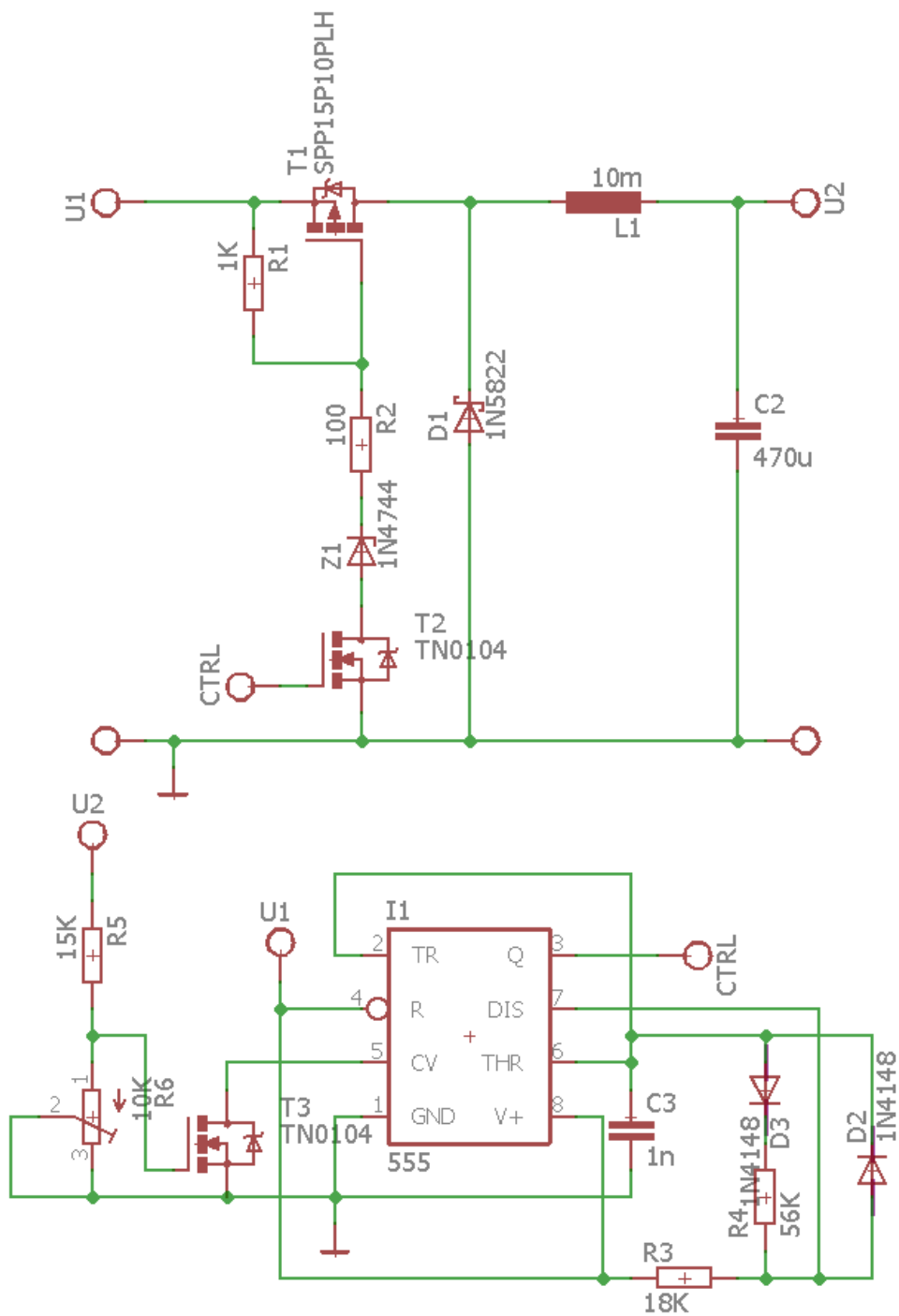
Obr. 18: Konkrétní zvyšující DC/DC měnič řízený obvodem 555
