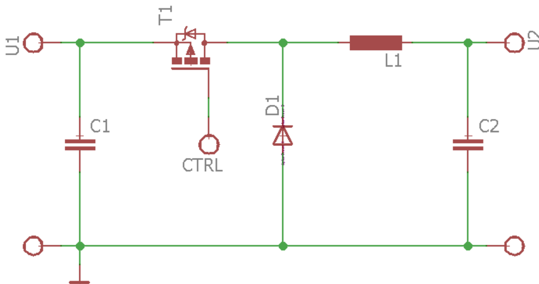
Obr. 6: Snížující měnič napětí
