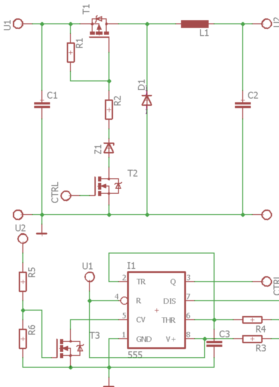
Obr. 7: Schéma DC/DC měniče s konverzí vstupního napětí dolů a obvodem 555
