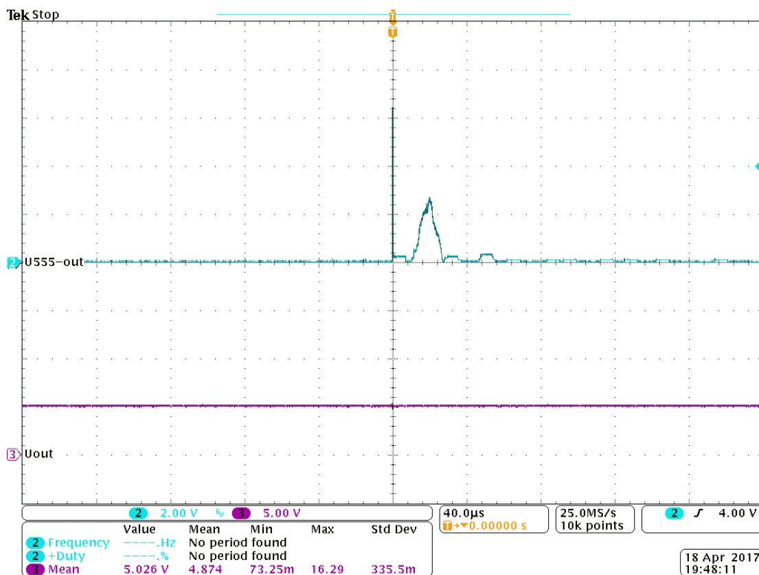
Obr. 19: Časové průběhy spínacího signálu (zeleně) a výstupního napětí (fialově) nezátíženého snižujícího měniče s obvodem 555
