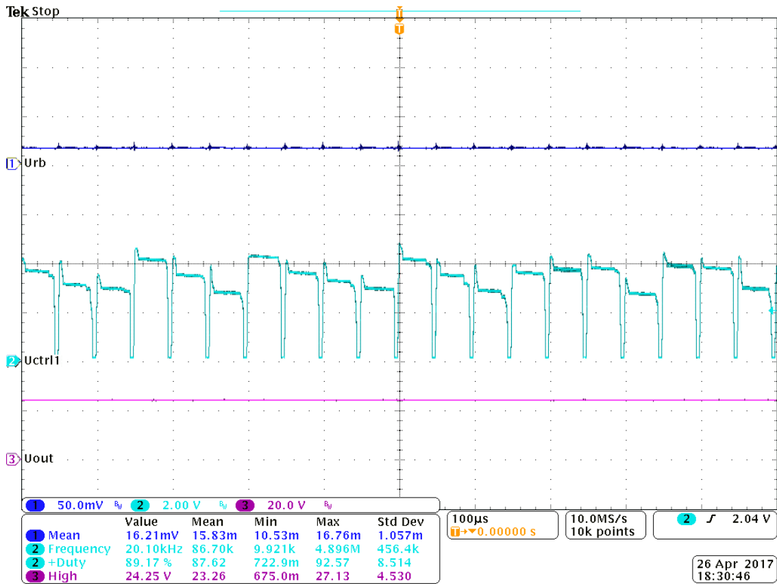
Obr. 40: Časové průběhy proudu (modře), spínacího signálu (zeleně) a výstupního napětí (fialově) zvyšujícího zatíženého měniče – zátěž 4,7 k \Omega
