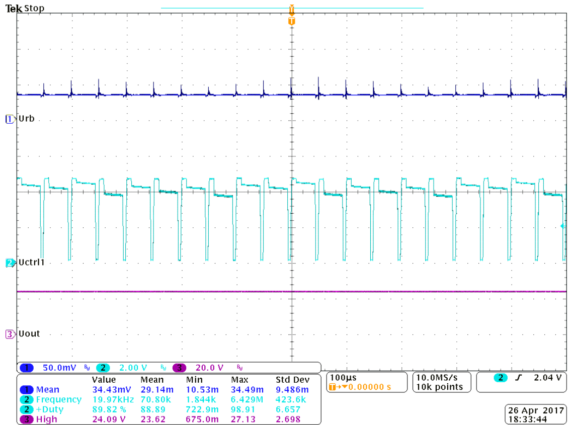
Obr. 41: Časové průběhy proudu (modře) spínacího signálu (zeleně) a výstupního napětí (fialově) zvyšujícího zatíženého měniče – zátěž 1 k \Omega
