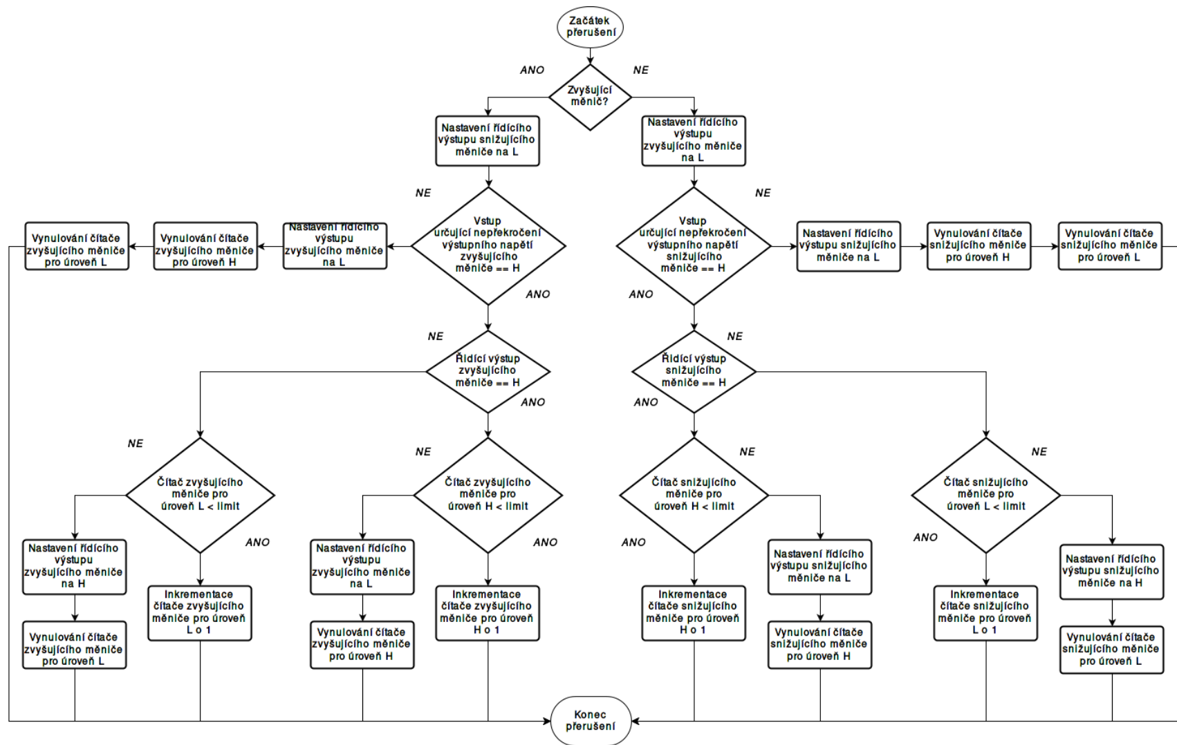
Obr. 28: Vývojový diagram obsluhy přerušení ukázkového programu pro obousměrný DC/DC měnič
