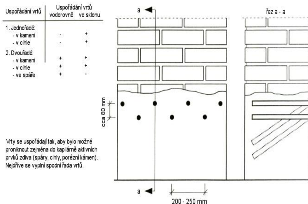
Obr. 12 – Tlaková injektáž [18]
