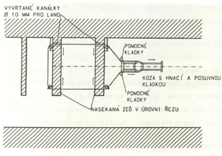
Obr. 8 – Schéma lanové pily [9]
