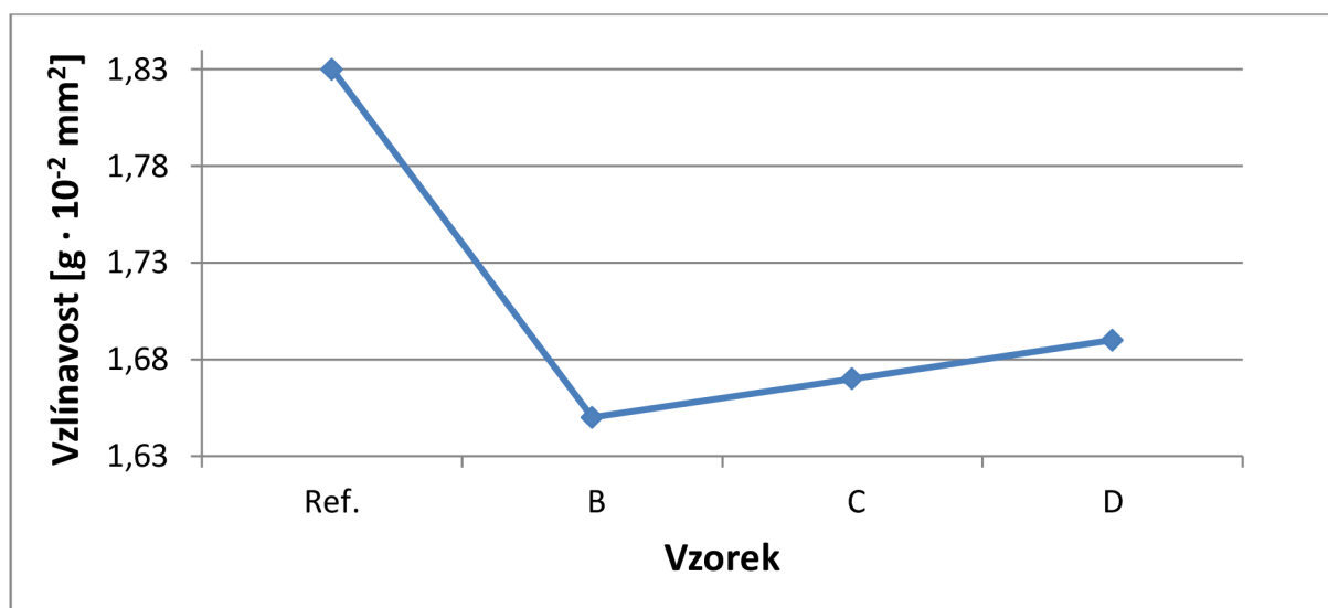
Obr. 24 – Výsledky stanovení vzlínavosti smíšeného zdiva
