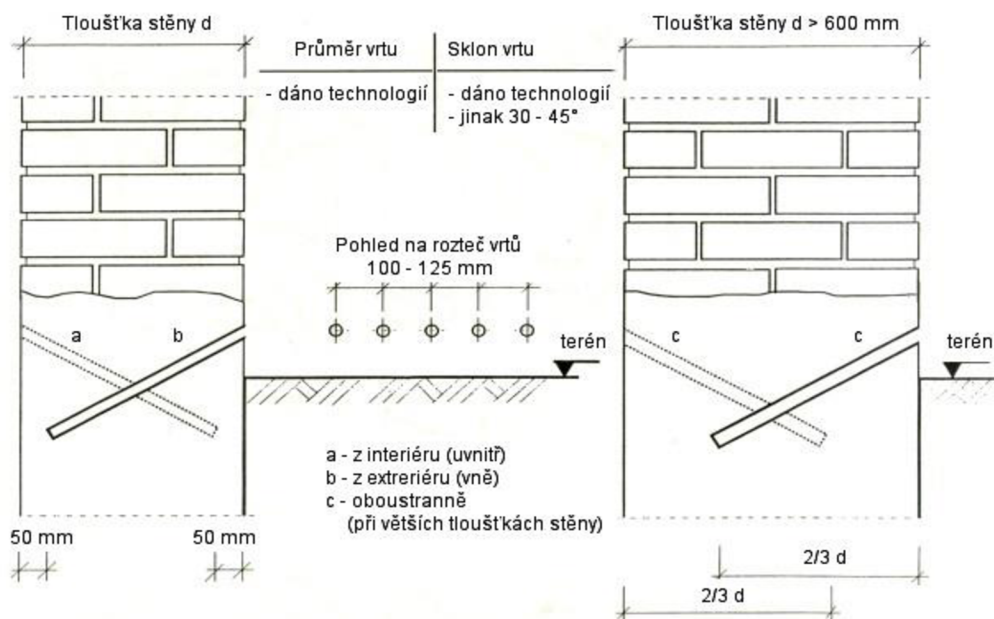
Obr. 11 – Beztlaková injektáž [18]
