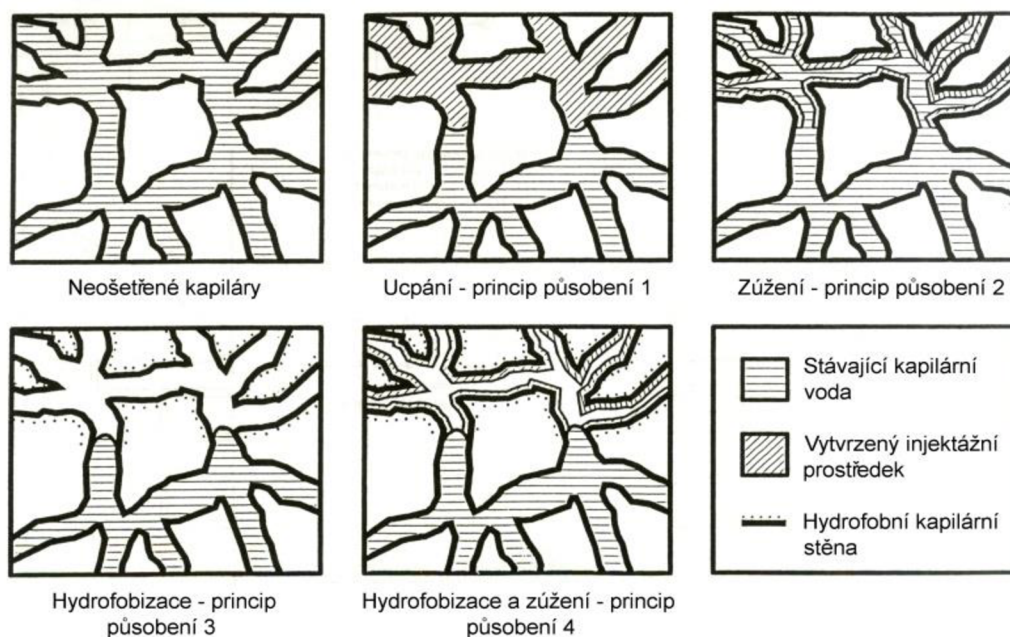
Obr. 13 – Principy působení snižování vlhkosti – schematické zobrazení [18]
