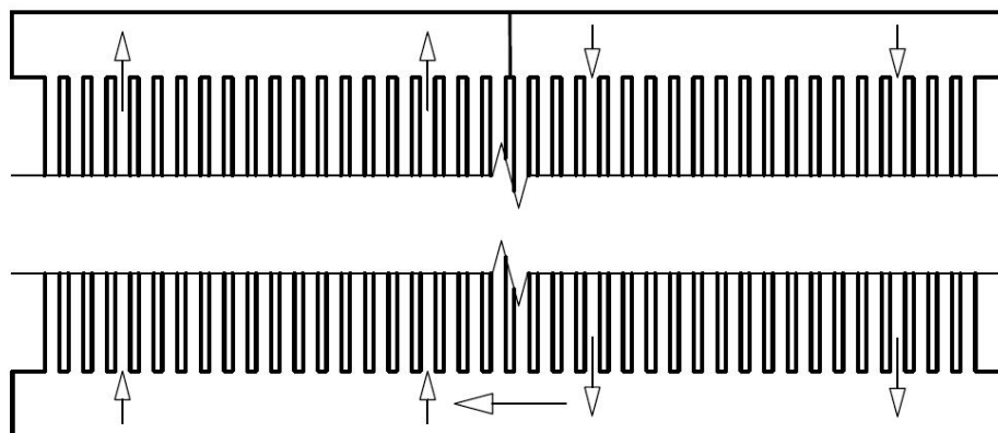
Obr. Chyba! V dokumentu není žádný text v zadaném stylu.. 10-2 Schématické znázornění proudění v membránové stěně PP1 na bocích tahu
