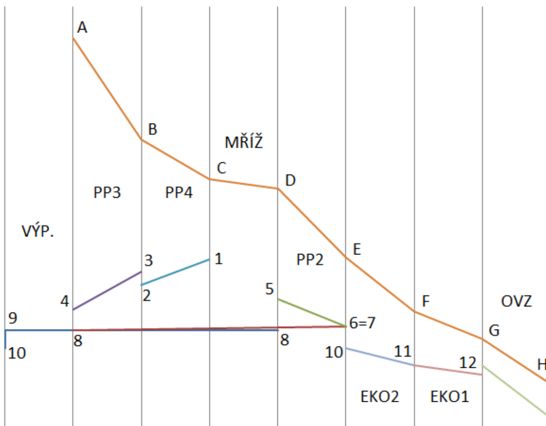
Obr. 6-1 Pilový diagram
