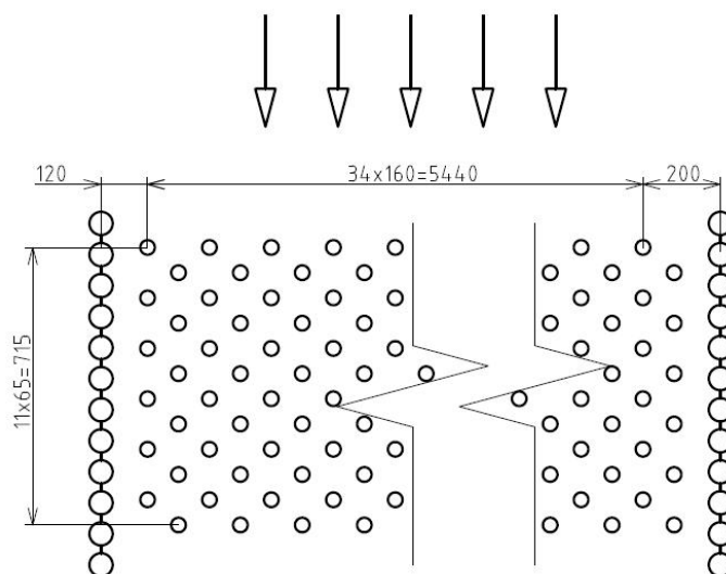
Obr. 8-1 Přehřívák 4
