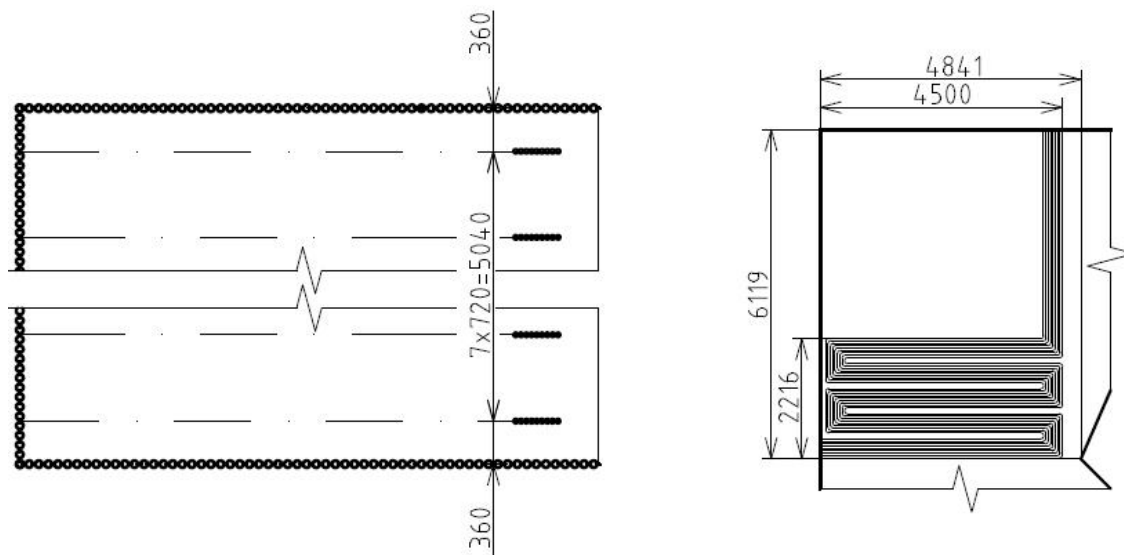
Obr. 7-1 Přejhřívák 3
