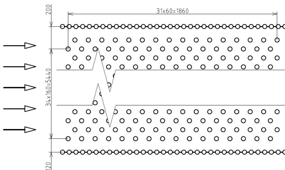
Obr. 10-1 Přehřívák 2
