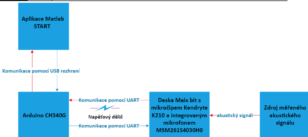
Obrázek 15 Navrhovaná konstrukce zařízení
