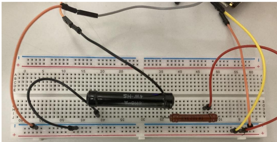
Obrázek 16 Napěťový dělič
