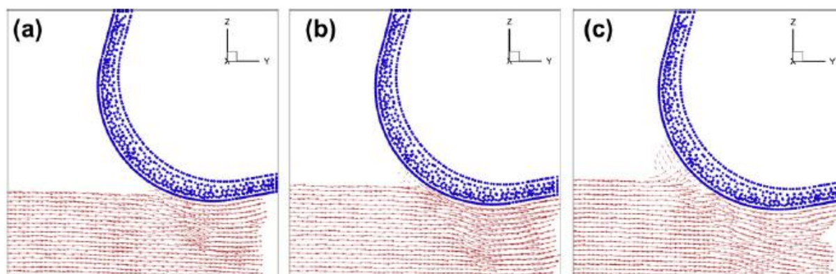
Obr. 38 Přebodový mechanismus od klouzání k řezání pro nástroj s poloměrem břitu 4,7 nm v malých hloubkách řezu, (a) 0,36 nm, (b) 0,72 nm, a (c) 1,09 nm [35].
