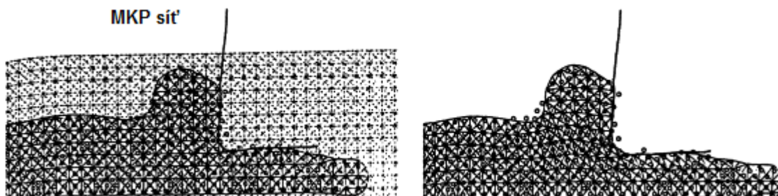
Obr. 34 Síť konečných prvků pro simulaci mikroobrábění [33].
