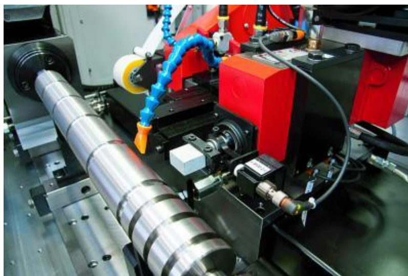
Obr. 28 Modulární systém obrábění [25].
