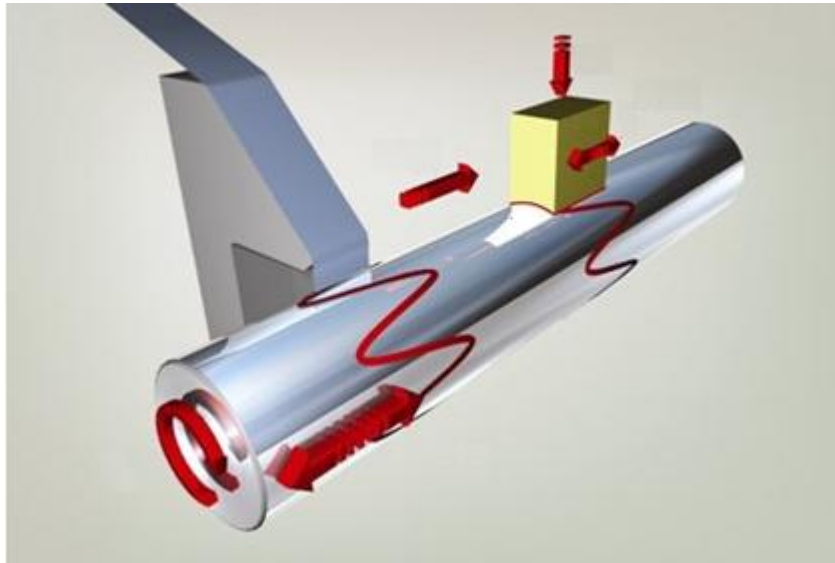
Obr. 23 Princip superfinašování [22].
