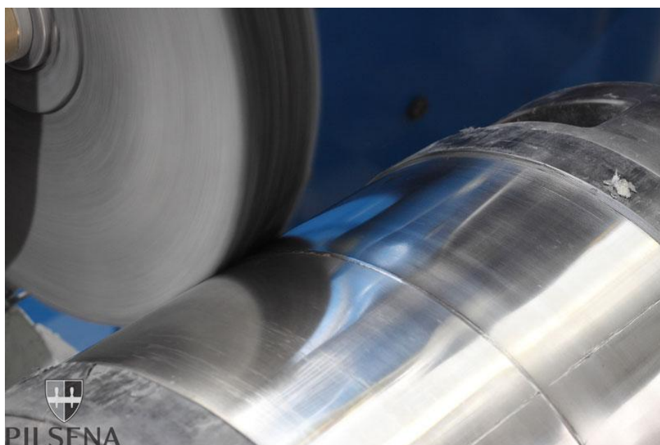
Obr. 30 Leštění válcové plochy pomocí leštícího kotouče [27].
