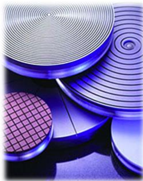
Obr. 18 Lapovací kotouče [19].
