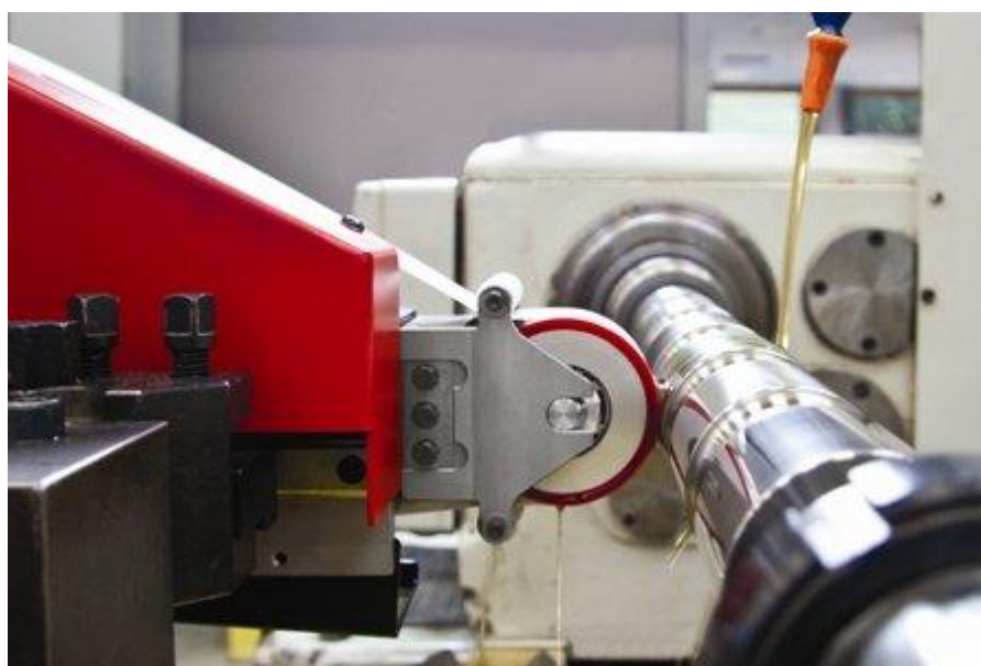
Obr. 25 Superfinašování superfinašovacím pásem s přítlačnou kladkou [22].
