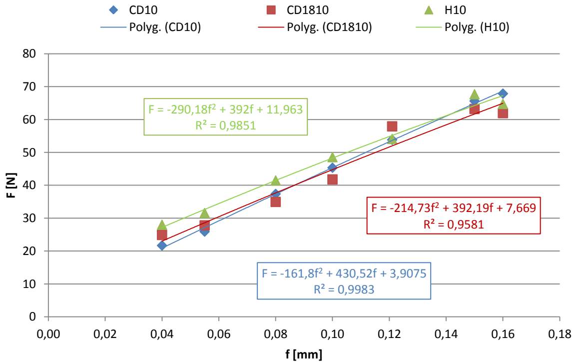
Obr. 65 Celkové síly pro řeznou rychlost 100 m/min.
