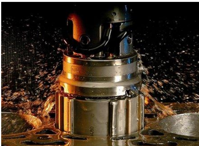
Obr. 15 Honovací hlava [16].
