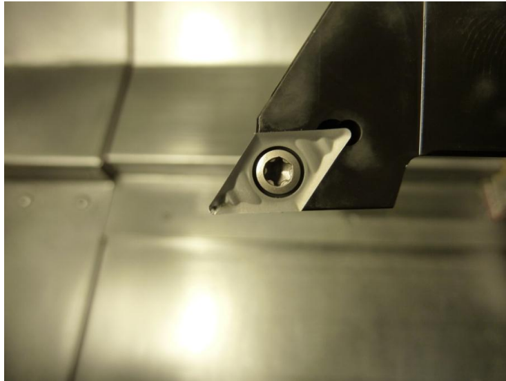
Obr. 41 Vyměnitelná břitová destička DCGX11T308-Al H10.
