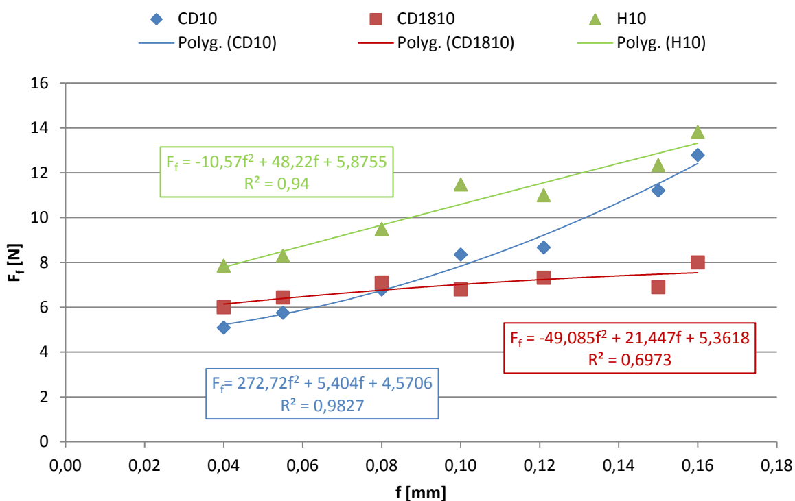
Obr. 58 Posuvové síly F_f při řezné rychlosti 200 m/min.
