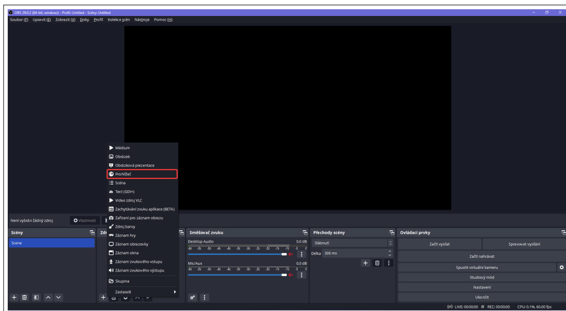
Obrázek 17: Vybrání zdroje
