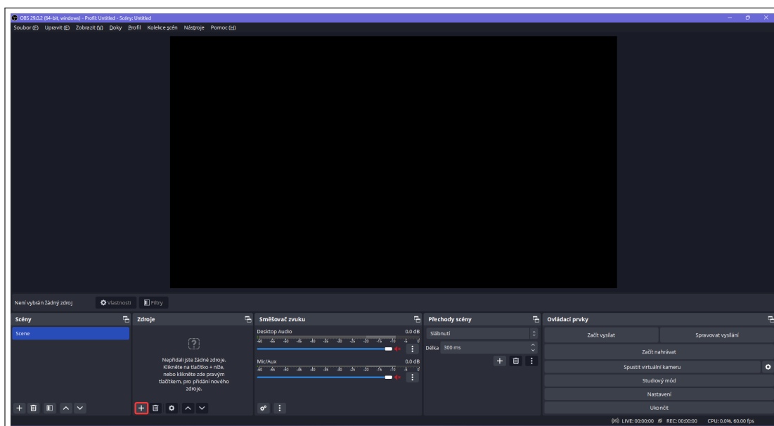
Obrázek 16: Vytvoření zdroje
