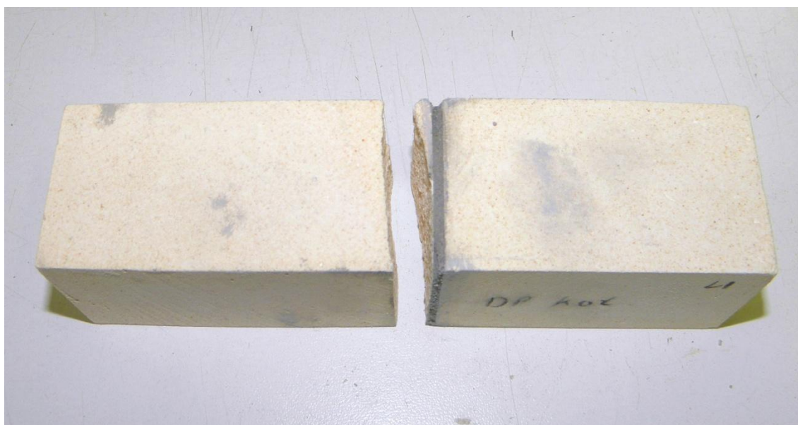
Obr. 7.1: Porušení zkušebního tělesa mimo tmel
