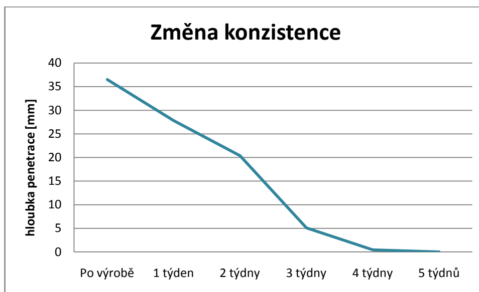
Graf 8.8: změna konzistence – tmel bez dietylenglykolu
