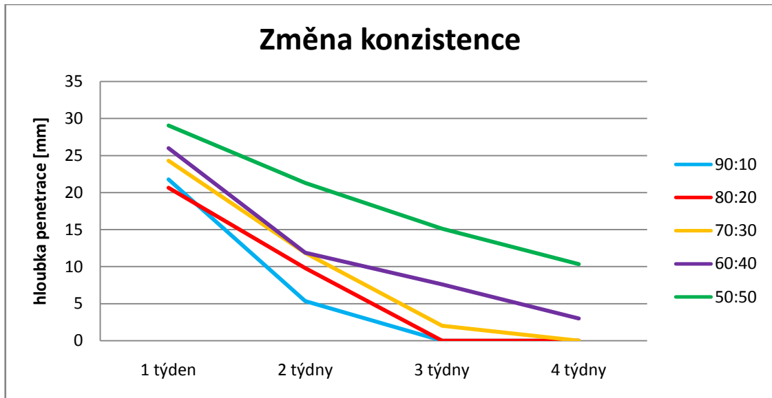
Graf 8.6: porovnání změny konzistence všech tmelů
