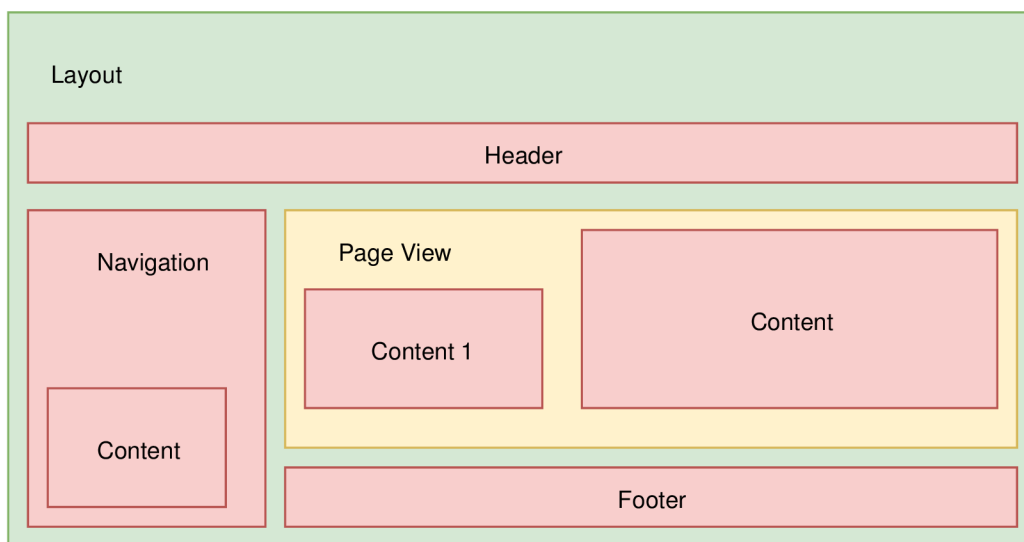
Obr. 3.3: Príklad rozloženia webovej stránky a rozdelenie jej častí do troch tried, zeleňá : rozloženie stránky ( Layout ), žltá : hlavný obsah stránky ( View ), červená : opakovateľné časti stránky ( Subview ).
