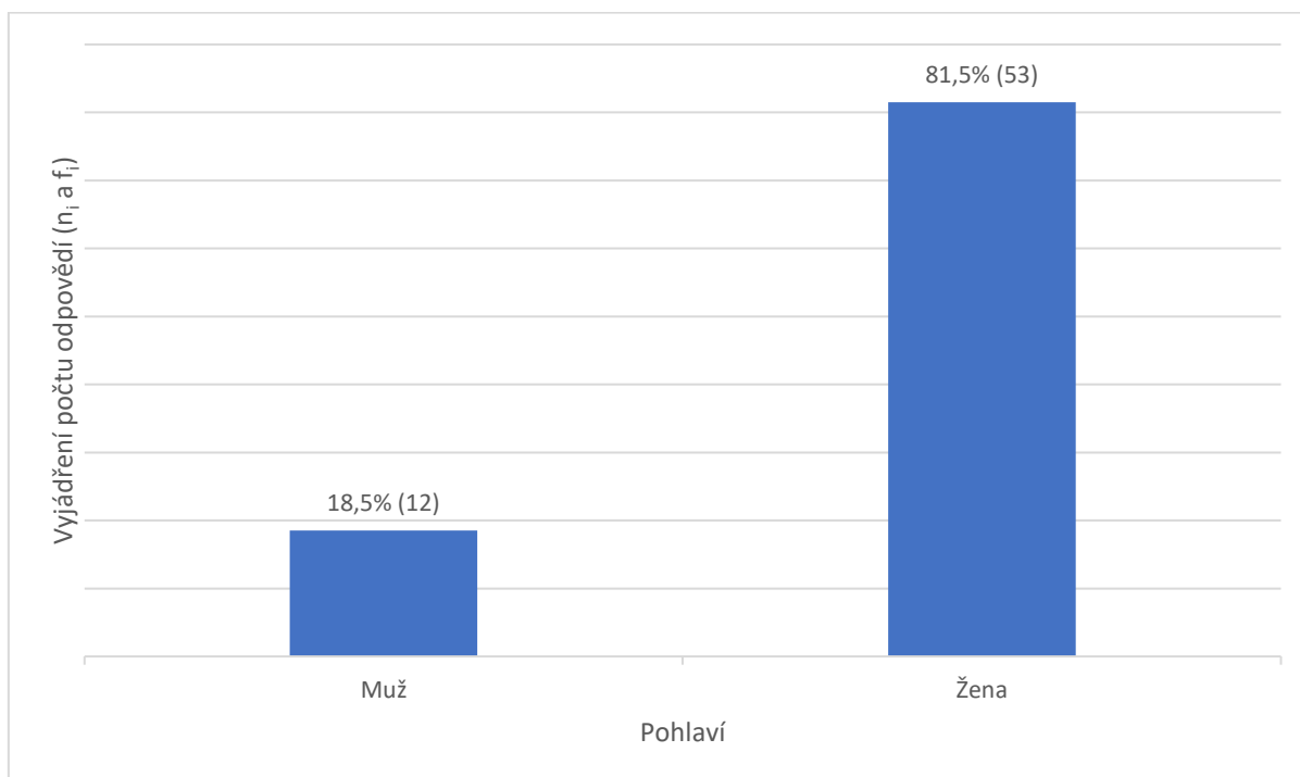
Graf č. 1: absolutní ( n_i ) a relativní četnost ( f_i ) odpovědí na položku č. 1
