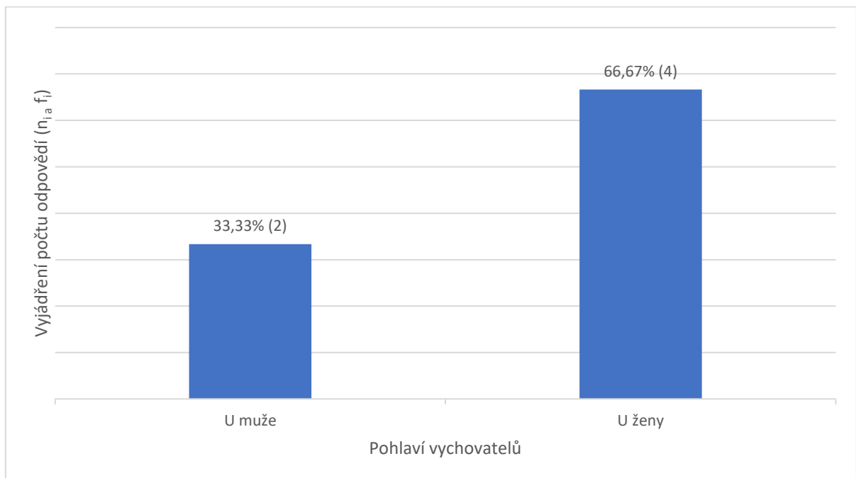
Graf č. 6: absolutní ( n_i ) a relativní četnost ( f_i ) odpovědí na položku č. 10 (dle zadání, n=6 )
