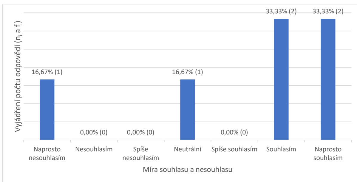
Graf č. 8: absolutní ( n_i ) a relativní četnost ( f_i ) odpovědí na položku č. 19 (dle zadání, n=6 )
