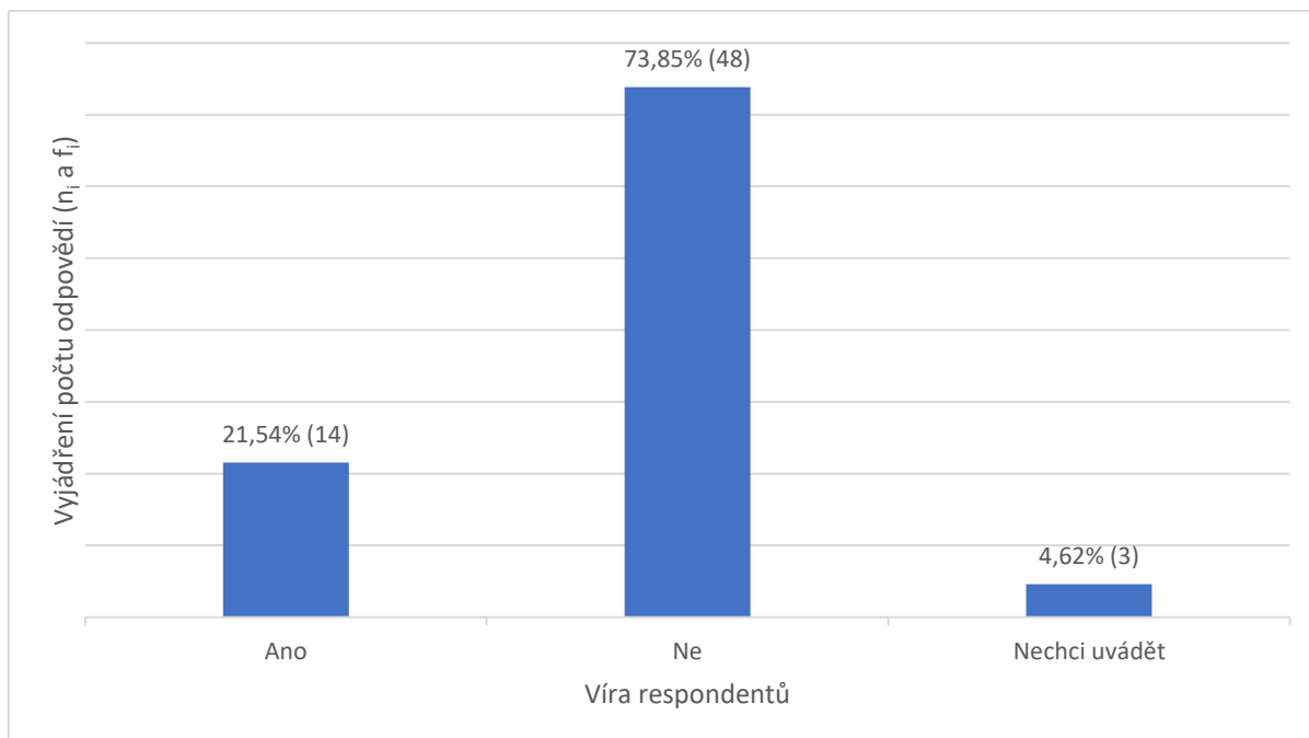
Graf č. 3: absolutní ( n_i ) a relativní četnost ( f_i ) odpovědí na položku č. 3
