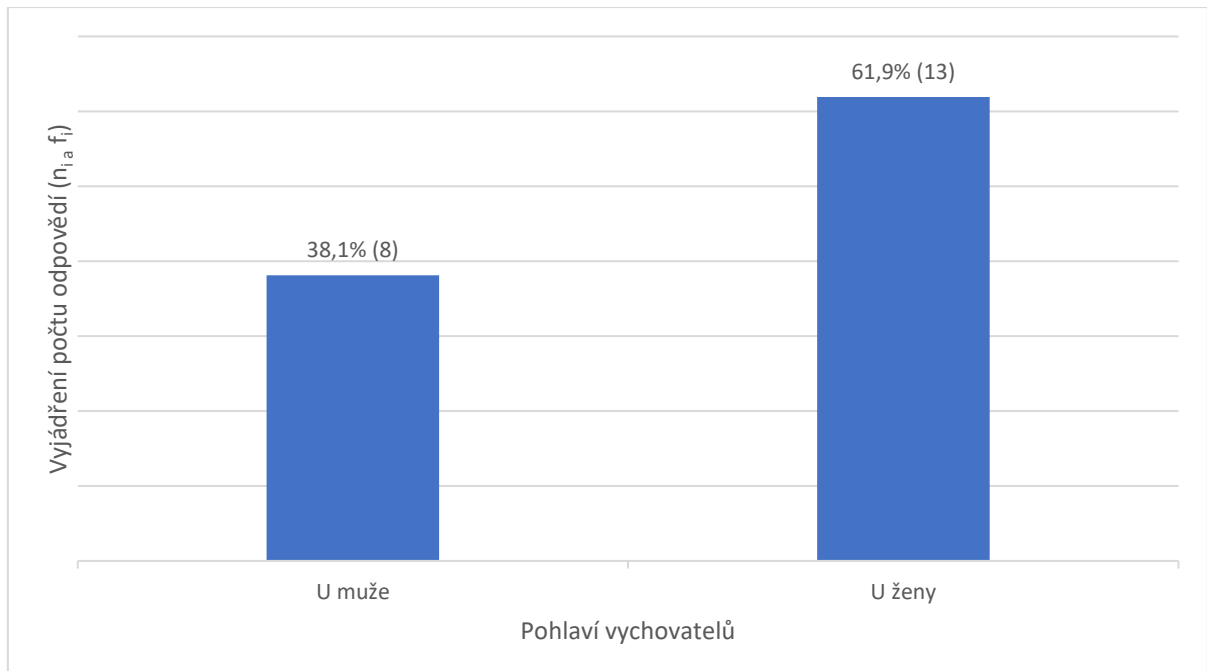
Graf č. 7: absolutní ( n_i ) a relativní četnost ( f_i ) odpovědí na položku č. 10 (celkem, n=21 )
