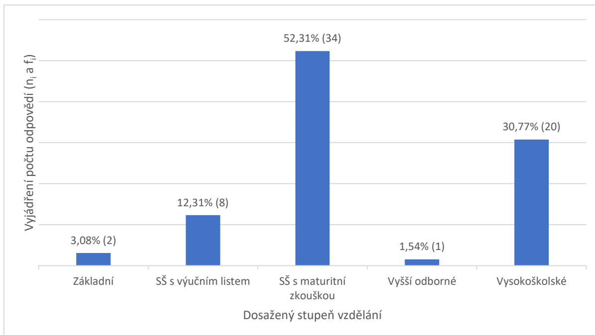
Graf č. 4: absolutní ( n_i ) a relativní četnost ( f_i ) odpovědí na položku č. 4
