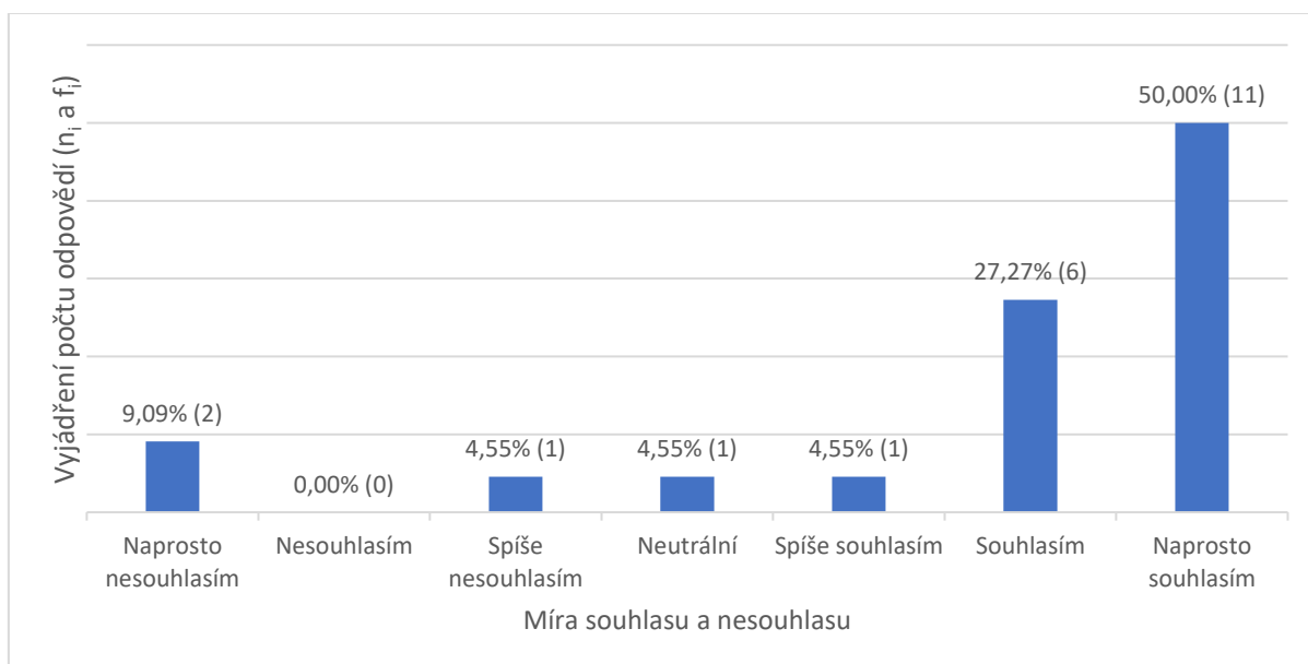
Graf č. 9: absolutní ( n_i ) a relativní četnost ( f_i ) odpovědí na položku č. 19 (celkem, n=22 )
