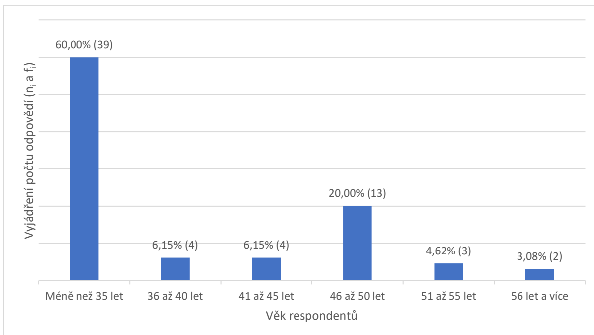
Graf č. 2: absolutní ( n_i ) a relativní četnost ( f_i ) odpovědí na položku č. 2
