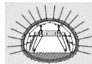
Finální obklad CIP betonem
