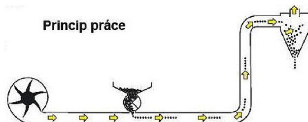
Obr. 1.9 Princip pneumatické dopravy
