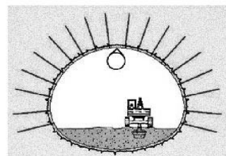
Bagrování dna (chystání na betonování)
