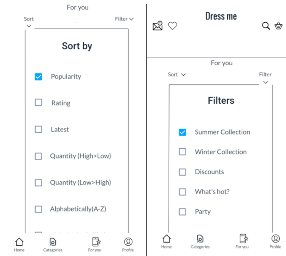
Obrázek 17-Grafický design-Stránky s roztříděním a filtrováním
