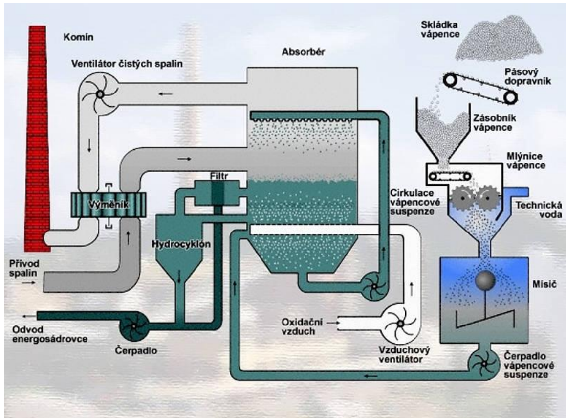
Obr. 3.10 Schéma mokré vápencové vypírky [13]
