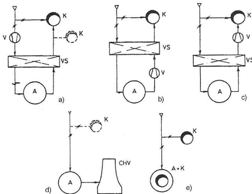
Obr. 3.12 Zjednodušená schémata odsiření mokrou vápencovou vypírkou V – spalínový ventilátor, K – komín, A – absorbér, VS – výměník spaliny/spaliny, CHV, – chladicí věž [2]
