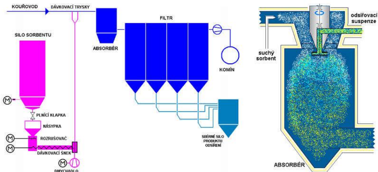
Obr. 3.9 Schéma souběžného odsiřování [11]
