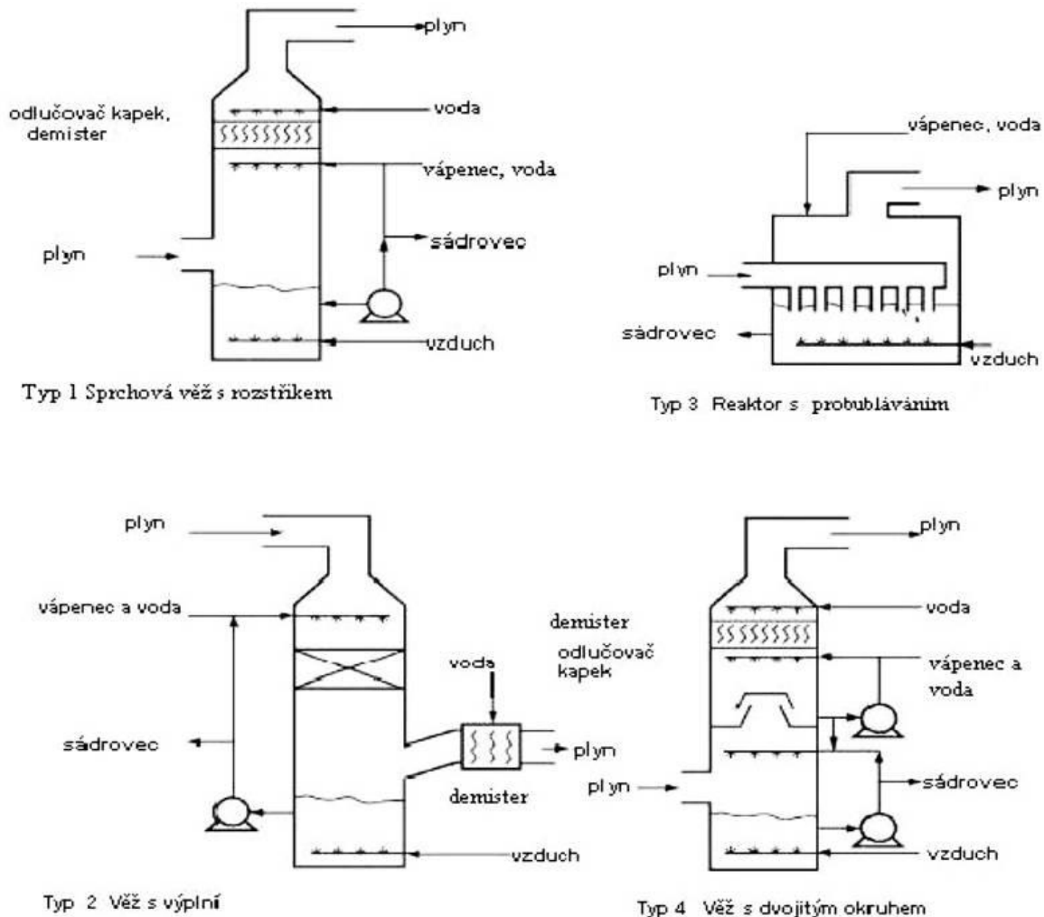
Obr. 3.11 Typy absorbérů [3]
