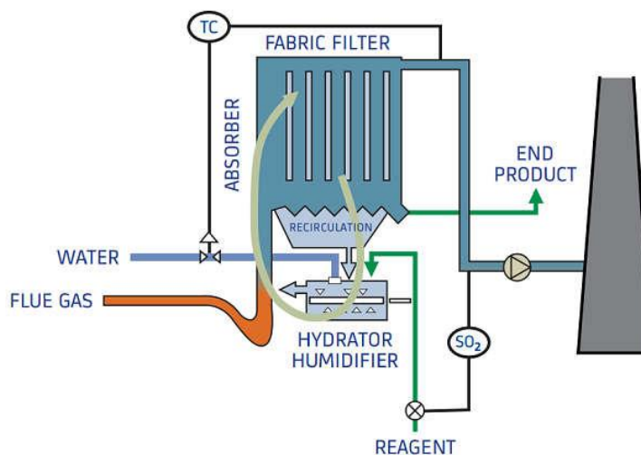
SYSTÉM RECIRKULACE
