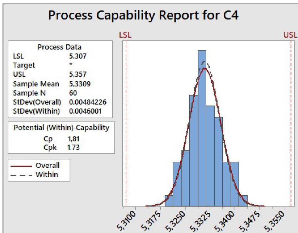
Obrázek 16: Způsobnost procesu (Zdroj: vlastní zpracování)
