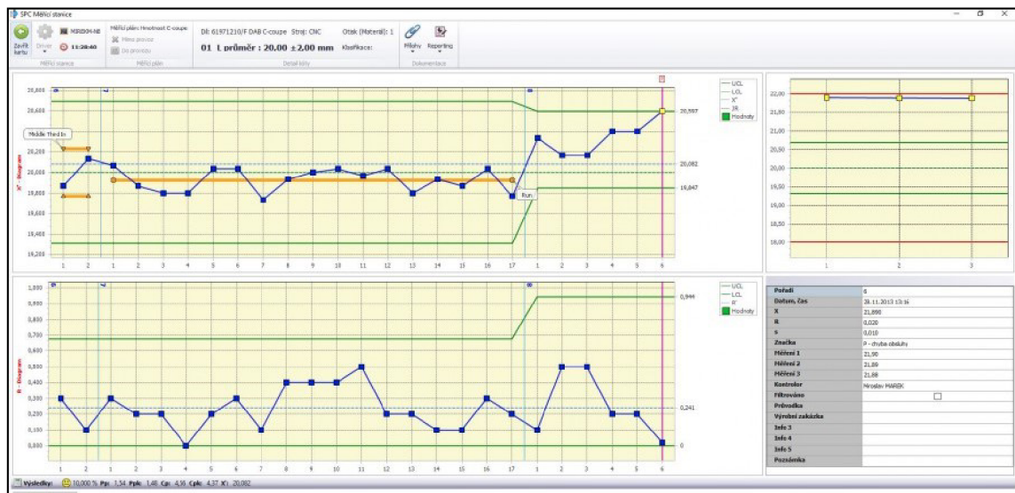
Obrázek 18: Modul SPC-měřící stanice (Zdroj: www.palstat.cz )
