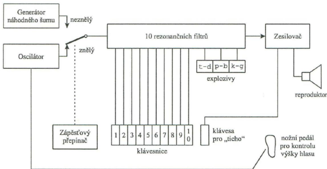
Obr. 1.2: Blokové schéma The Voder [7]
