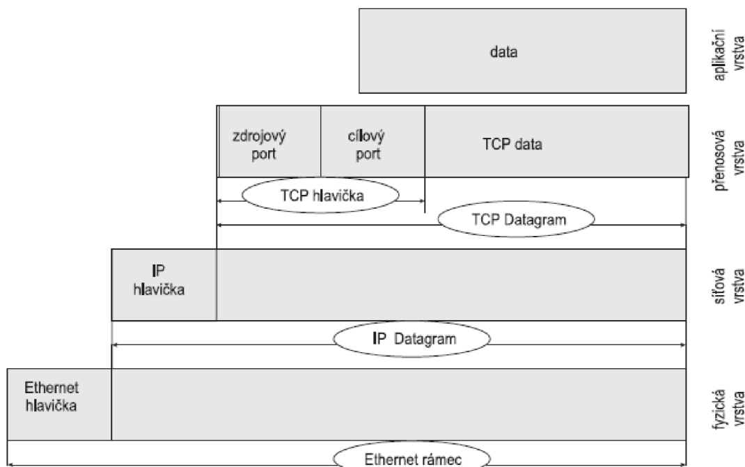
Obrázek 1 - Schéma vrstev protokolu TCP/IP
