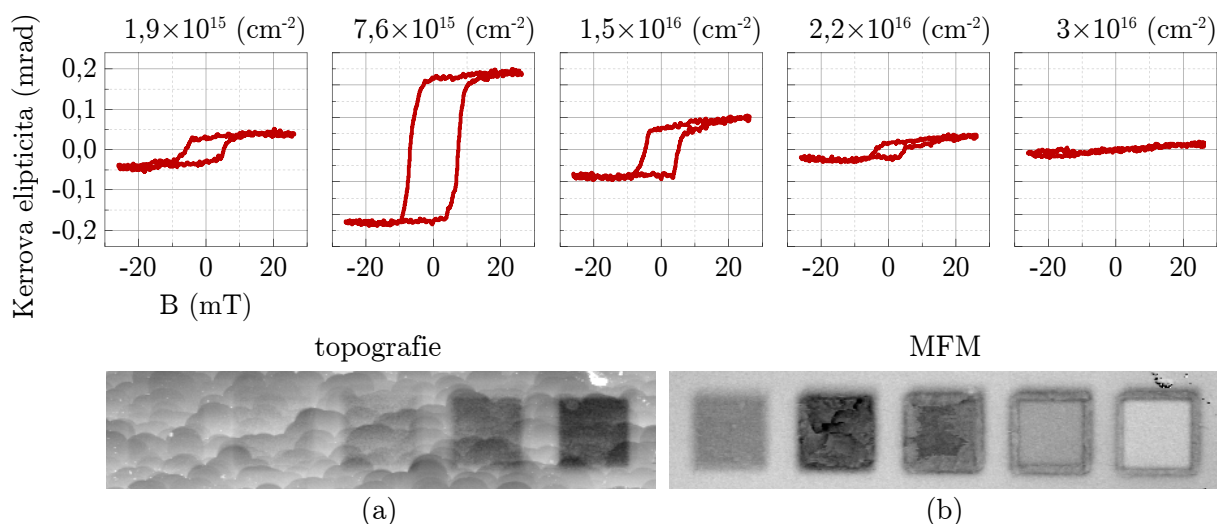
Obr. 5.1: Struktury o hraně 3 \mu\text{m} transformované zvyšující se (zleva) iontovou dávkou. Hysterézní smyčky Kerrové elipticity úměrné rovinné složce vektoru magnetizace byly měřeny pomocí MOKE v longitudinální konfiguraci. V dolní části obrázku je (a) topografie struktur a (b) fáze měřená MFM, ve které lze u struktur transformovaných dávkami 7,6 a 1,5 \times 10^{15} iontů/cm 2 vidět mikromagnetické uspořádání poukazující na propojení bcc krystalitů a transformaci celé ozářené oblasti.
