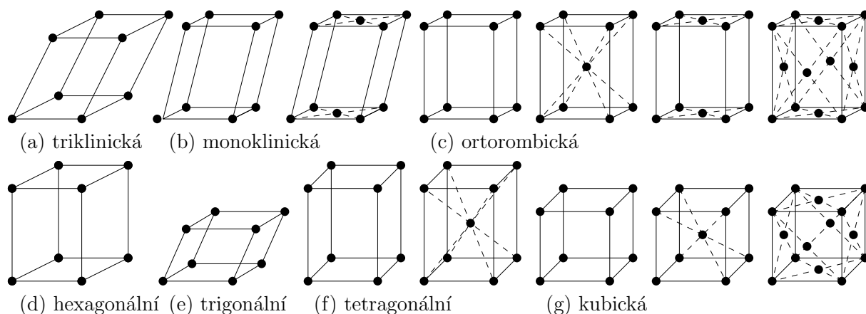
Obr. 1.2: Mřížky třídimenzionálních krystalových soustav.
