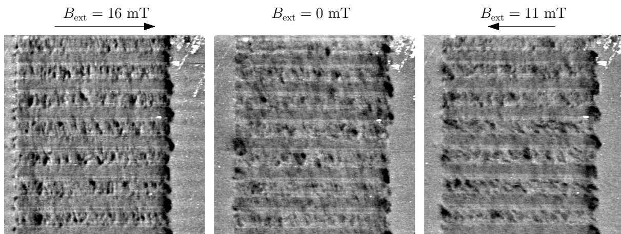
Obr. 6.9: Magnetické proužky o rozměrech 1,6 \mu\text{m} a 20 \mu\text{m} transformované střídavě dávkami 1,7 a 8,5 \times 10^{15} iontů/ \text{cm}^2 se zvyšující se vzájemnou vzdáleností od 200 nm do 500 nm. Proužky jsou umístěny podél směru přítomného externího magnetického pole proměnné velikosti.
