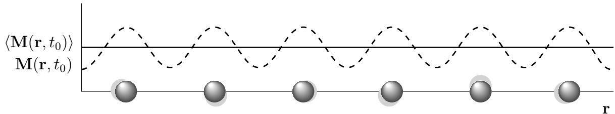
Obr. 2.1: Okamžitá lokální hustota magnetického momentu a její mezoskopický objemový a časový průměr ve schematickém znázornění jednodimenzionální atomární struktury.
