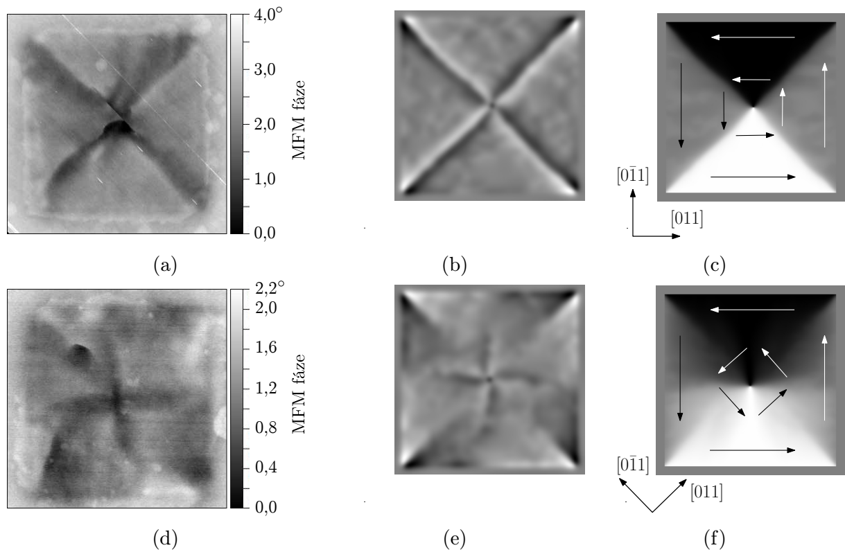
Obr. 6.3: Čtverce o hraně délky 1\ \mu\text{m} transformované dávkou 8 \times 10^{15} iontů/cm 2 a příslušné simulace magnetického stavu. Hrany struktur byly orientovány podél směru krystalových teras (a) – (c) a diagonálně vůči nim (d) – (f). Data (a) a (d) byla získána měřením fáze MFM, zatímco (b) a (e) simulací MFM v programu mumax 3 . Při simulaci jsme vycházeli z modelu složené čtyřčetné a uniaxiální anizotropie v zrnech čtyř krystalograficky významných orientací. Spolu se simulovanou x složkou vektoru magnetizace M_x jsou v (c) a (f) vyznačeny směry vektoru magnetizace \mathbf{M} v příslušných částech struktury.
