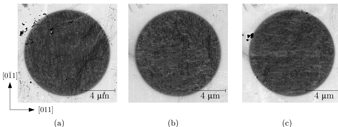
Obr. 5.2: SEM snímky disků o průměru 10 \mu\text{m} transformovaných shodnou dávkou iontů při rozdílných orientacích rastrování iontového svazku vůči krystalografickým terasám. Směr teras [0\bar{1}1] je na obr. orientován vertikálně a odchylky směr skenování jsou (a) 15^\circ , (b) 45^\circ a (c) 75^\circ .
