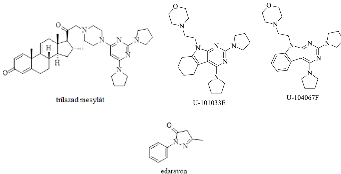
Obrázek 14 – vzorce lazaroidů
