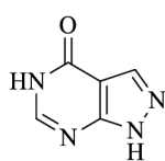
allopurinol
