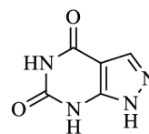
oxypurinol
