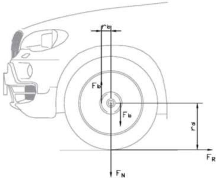
Obr. 2 - Znáznornění brzdne síly
