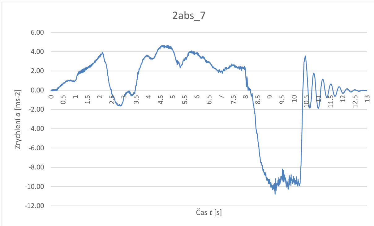
Graf č. 26 - Průběh zrychlení, 2abs_7
