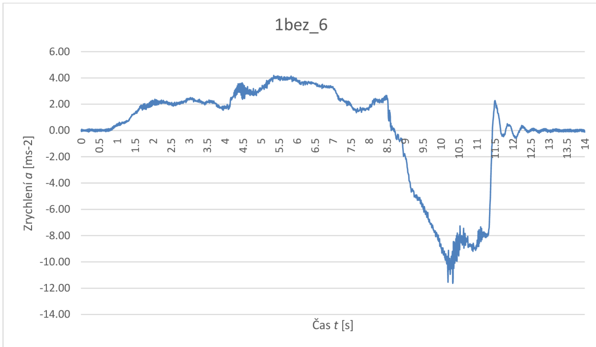
Graf č. 8 - Průběh zrychlení, 1bez_6
