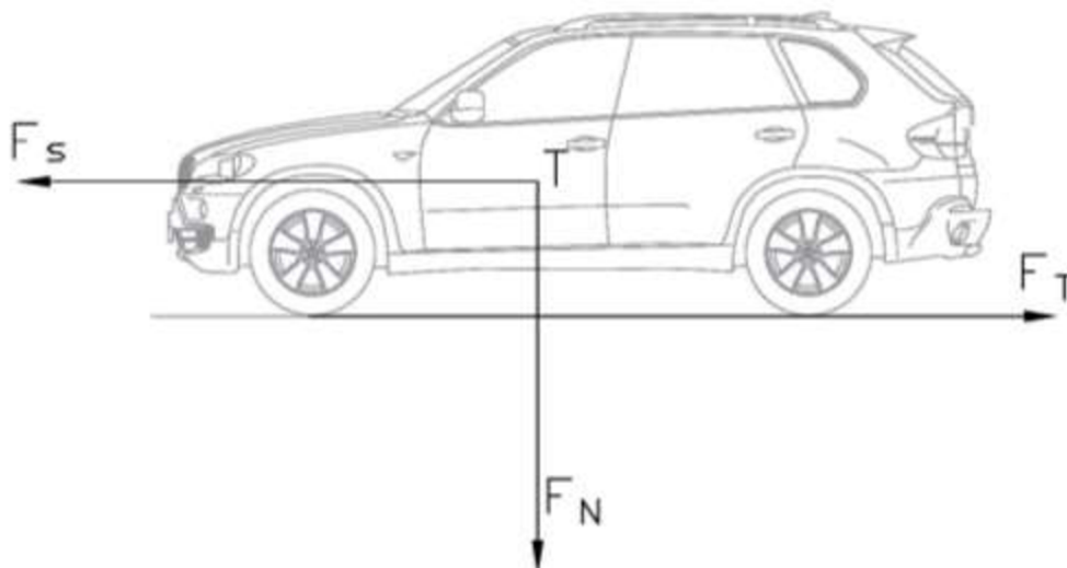
Obr. 1 - Znárodnění základních sil (třecí F_T ; normálová F_N ; setrvačná F_s )
