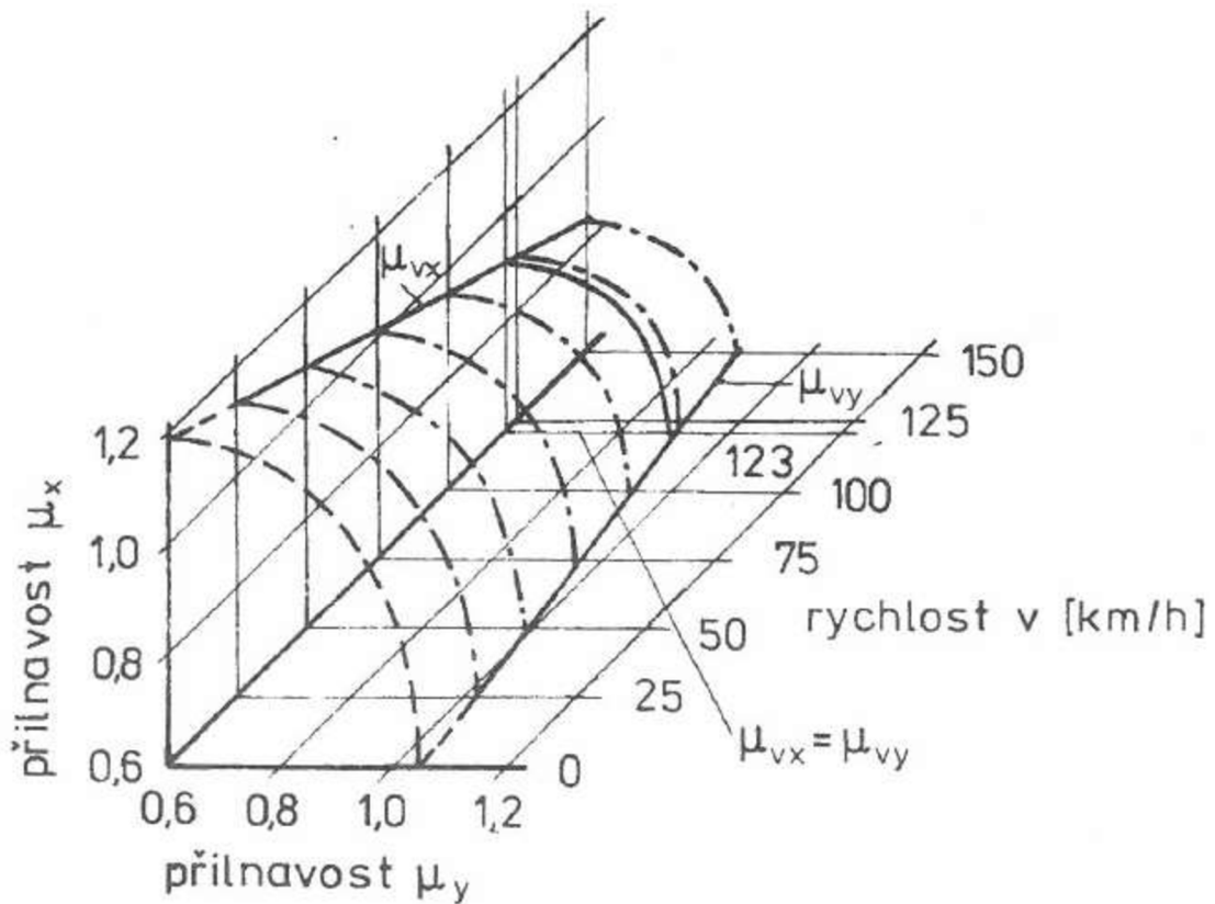
Graf č. 3 Tříosý průběh adheze v závislosti na rychlosti [2]
