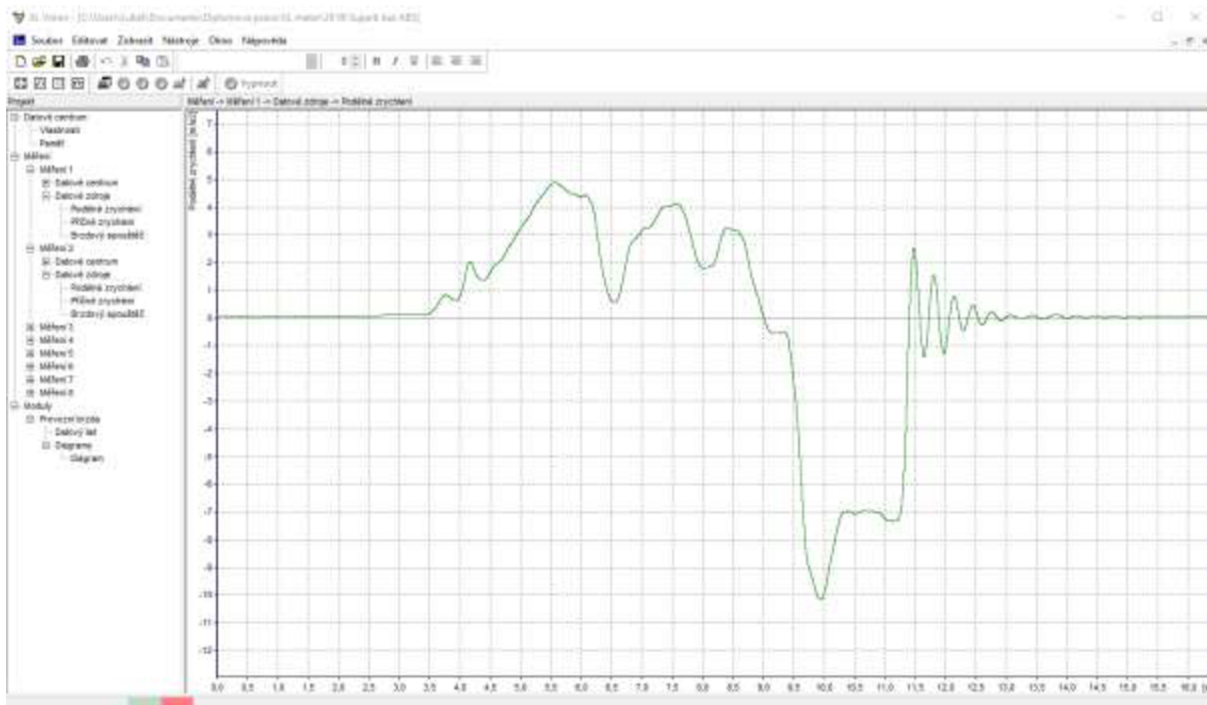
Obr. 24 Náhled na program XL Vision™, graf podélného zrychlení a zpomalení v čase
