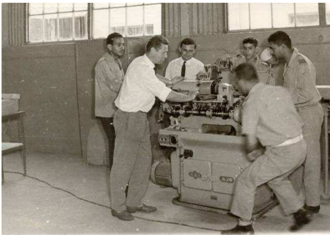
U československého automatického soustruhu A 20 – zleva řemeslník specialista Zaki, Oldřich Medřický, Ing. Jaroslav Rajlich a studenti 3. ročníku. (sbírka Ing. Jaroslava Rajlicha)
