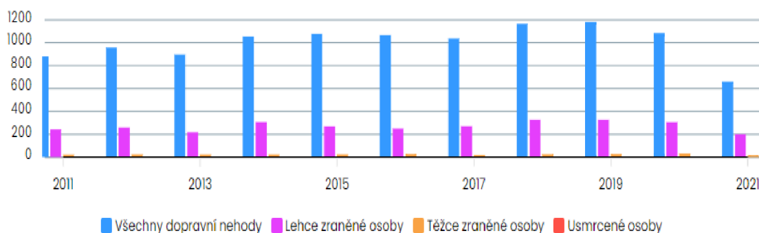
Obrázek 2: Graf dopravní nehodovosti na kruhových objezdech
