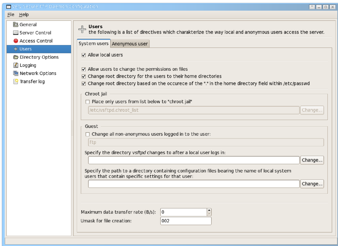
Obrázok 7.1: Výsledná aplikácia
