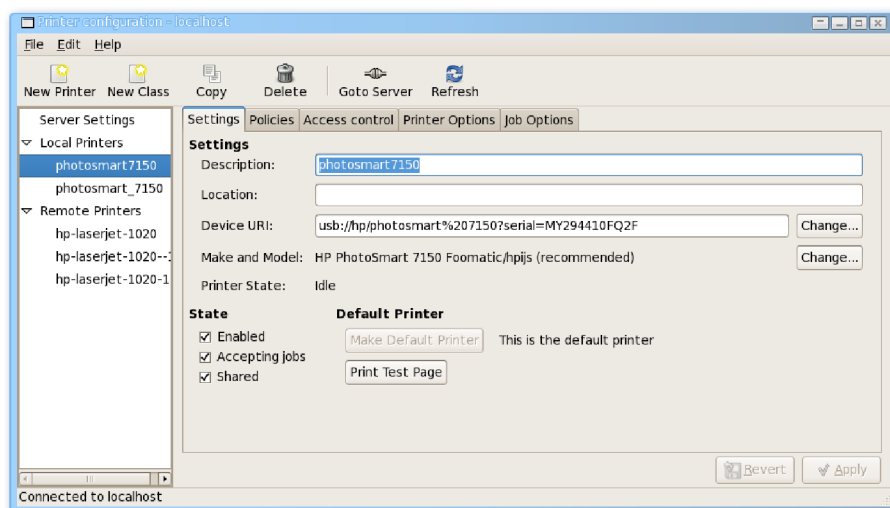
Obrázok 5.1: System-config-printer
