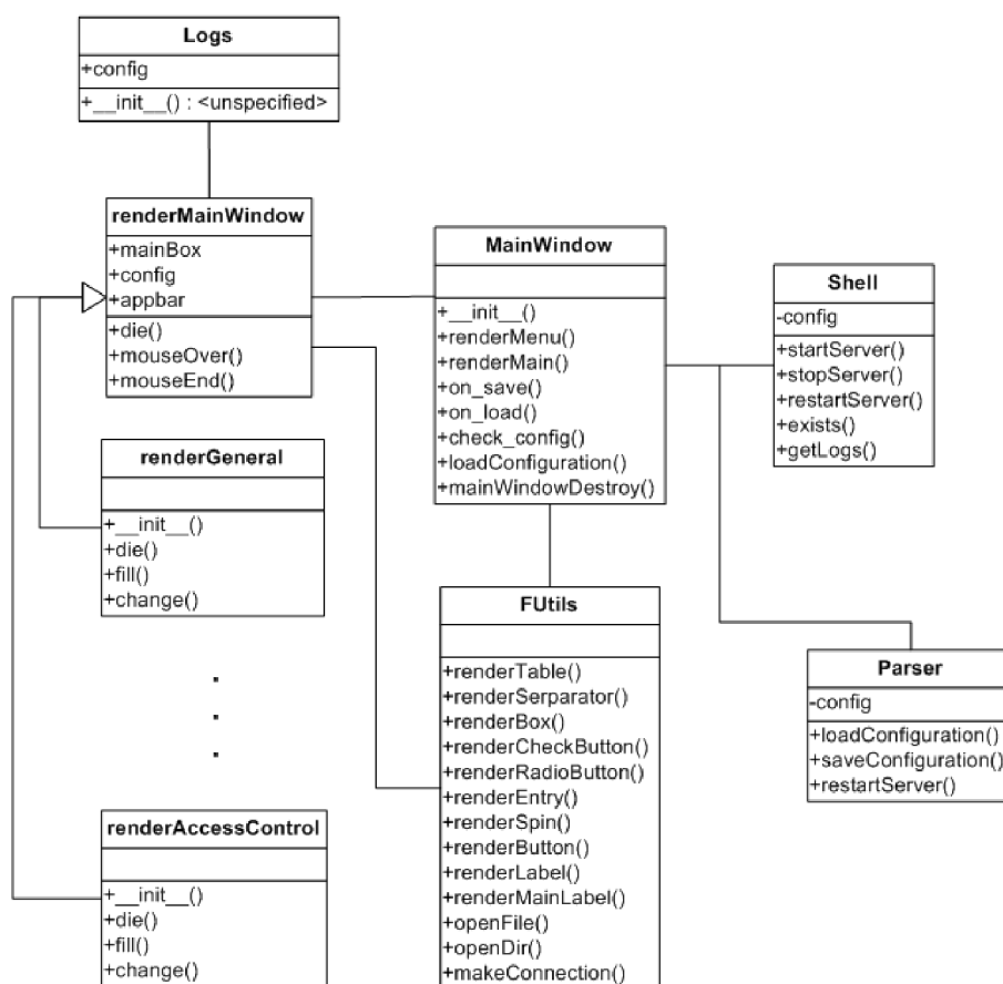
Obrázok 3.3: Diagram tried
