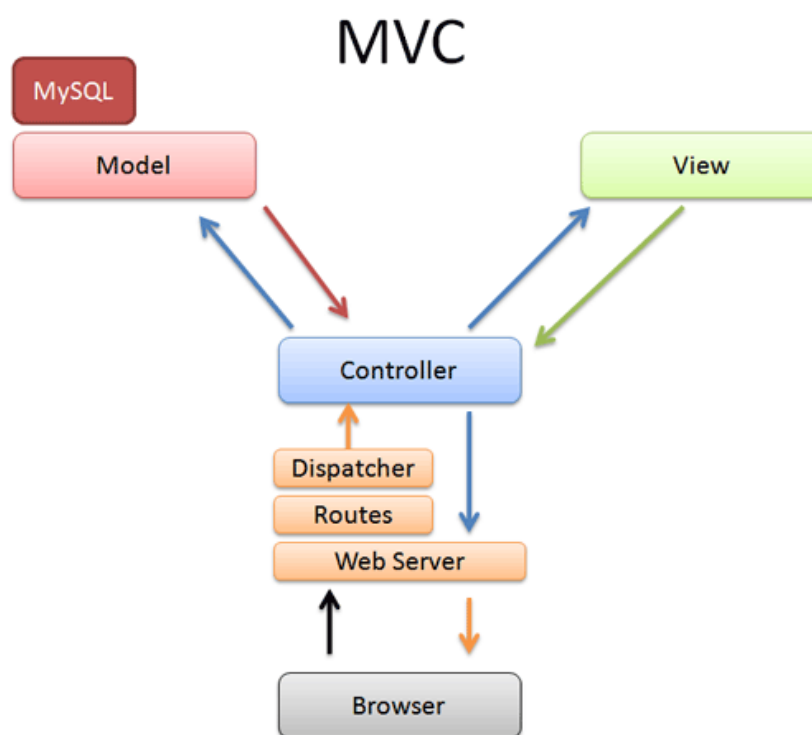
Obrázek 4.2: Návrhový model MVC
