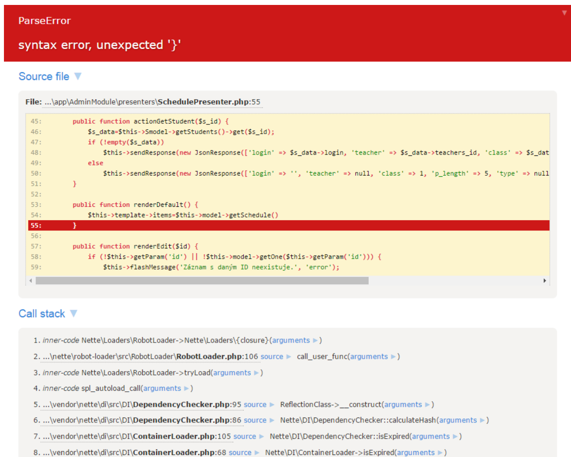
Obrázek 2.7: Diagnostický nástroj Tracy
