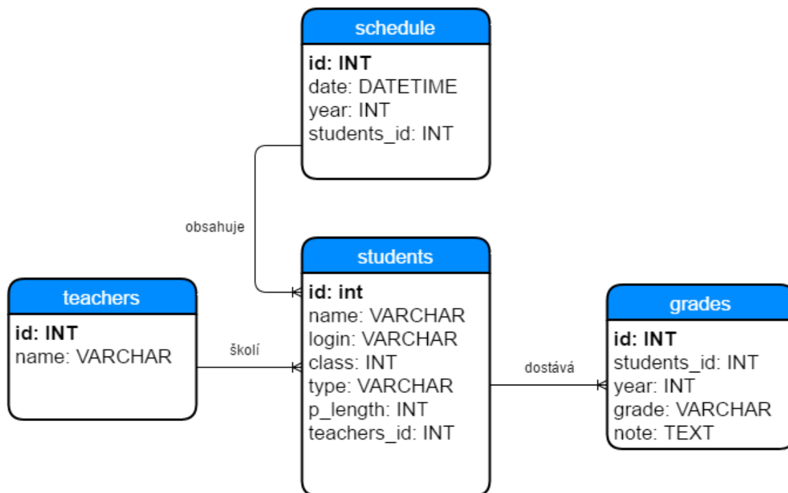
Obrázek 4.1: Entity-Relationship diagram
