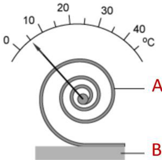
Obrázek 3 Bimetalový teploměr [7]
