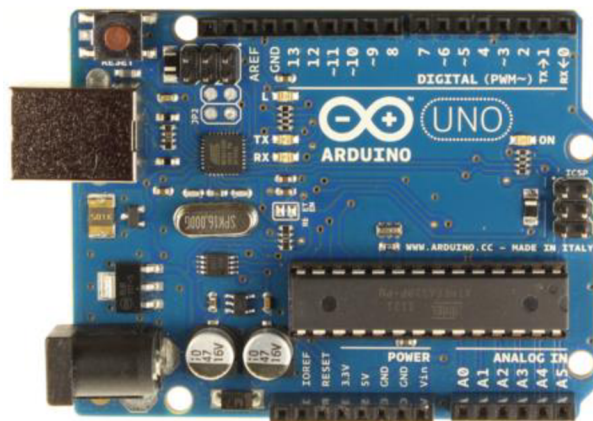
Obrázek 18 Arduino Uno [53]
