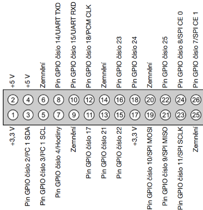
Obrázek 9 26pinový GPIO konektor [33]
