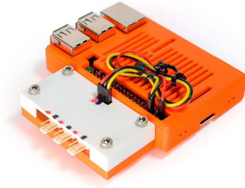
Obrázek 42 Zkompletované zařízení
