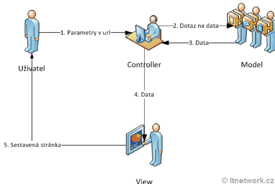
Obrázek 4 MVC architektura [18]
