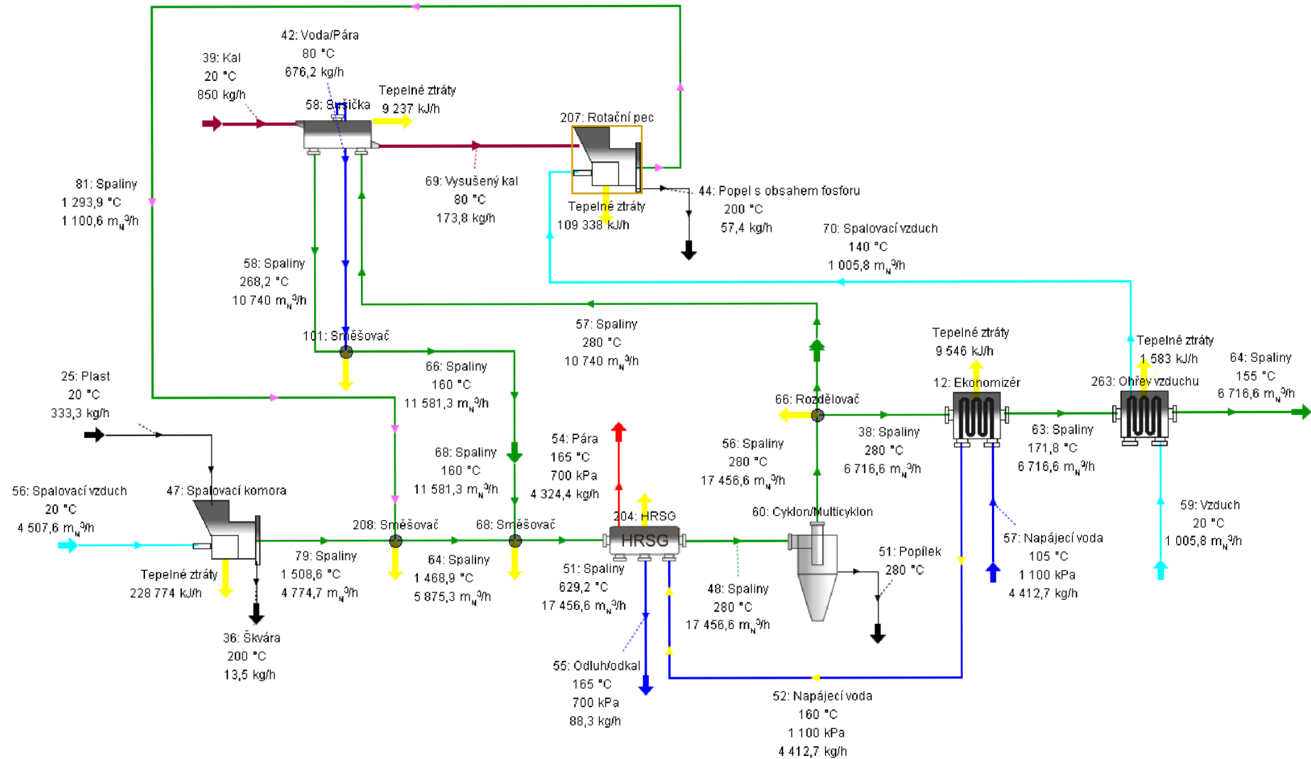
Obrázek 8.7 Schéma integrované technologie – varianta 2 (W2E)
