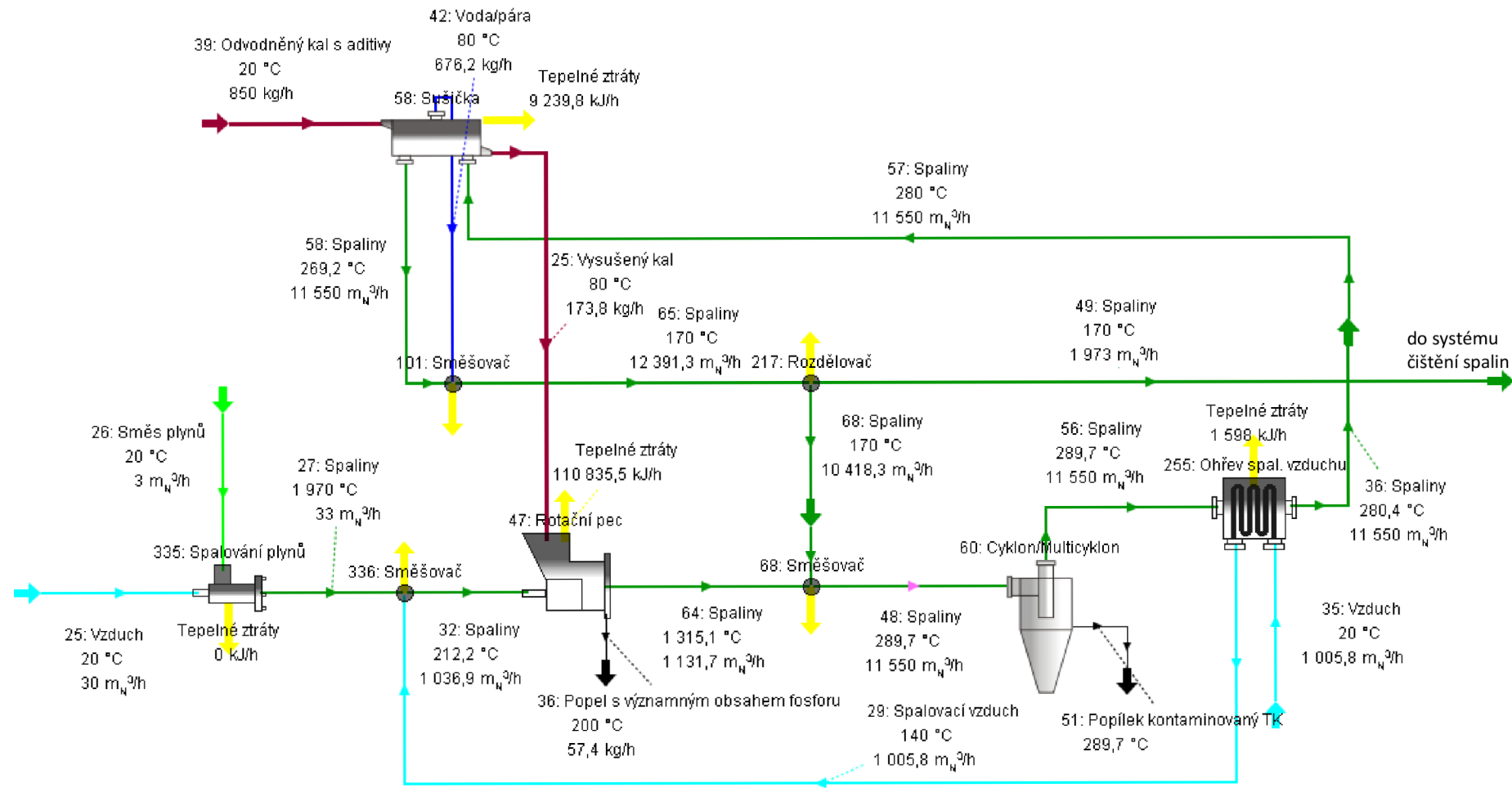
Obrázek 8.1 Schéma technologie zpracování kalů (W2E)
