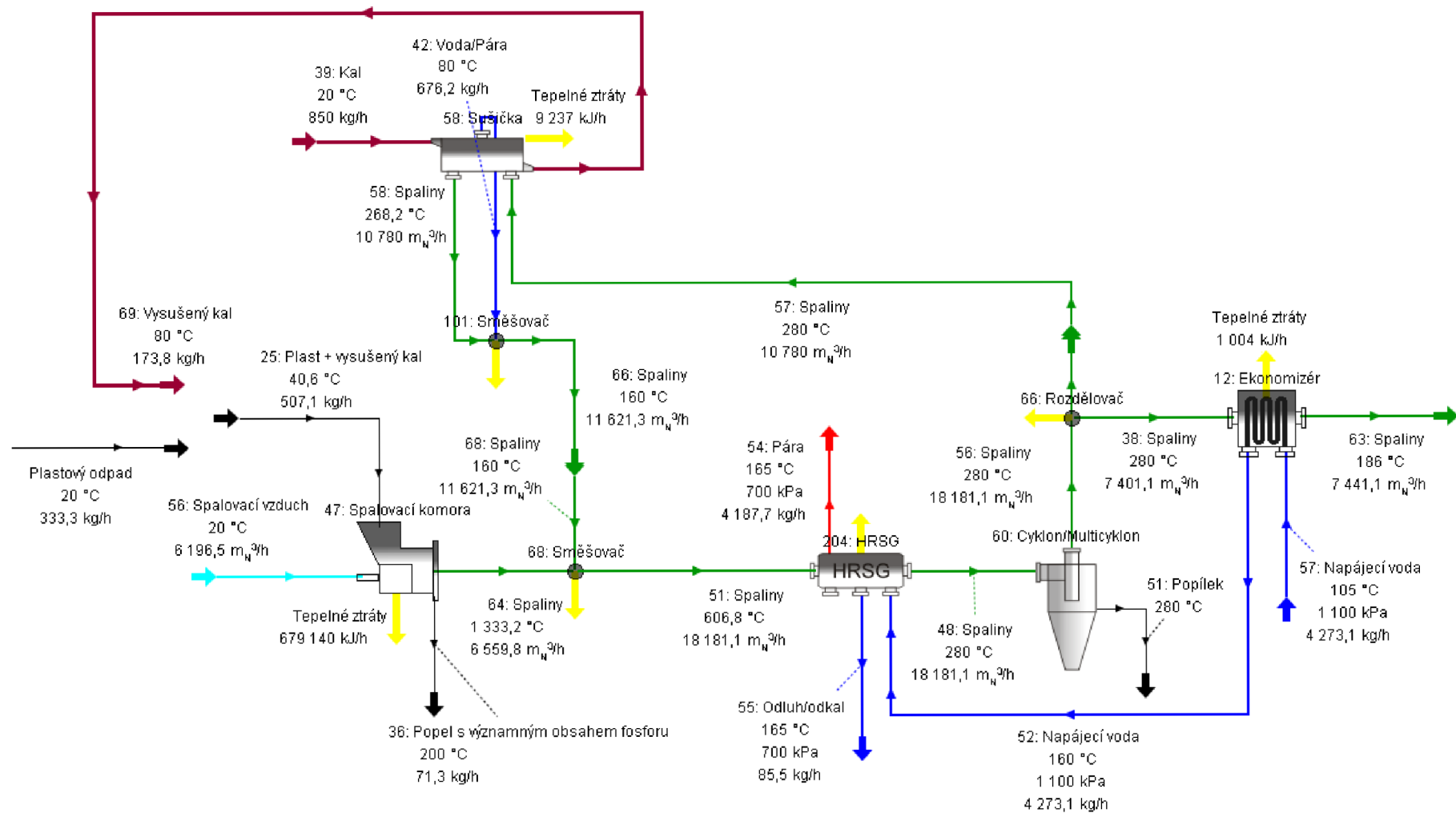
Obrázek 8.4 Schéma integrované technologie – varianta 3 (W2E)
