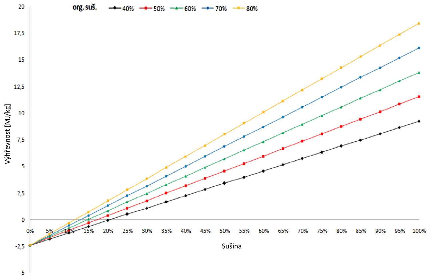
Obrázek 2.3 Závislost výhřevnosti kalu na obsahu sušiny a organické sušiny [7]
