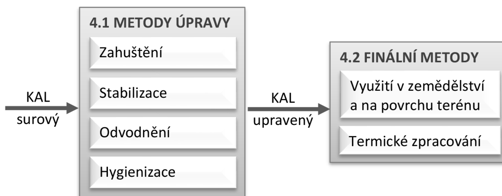
Obrázek 4.1 Metody úpravy a likvidace čistírenských kalů
