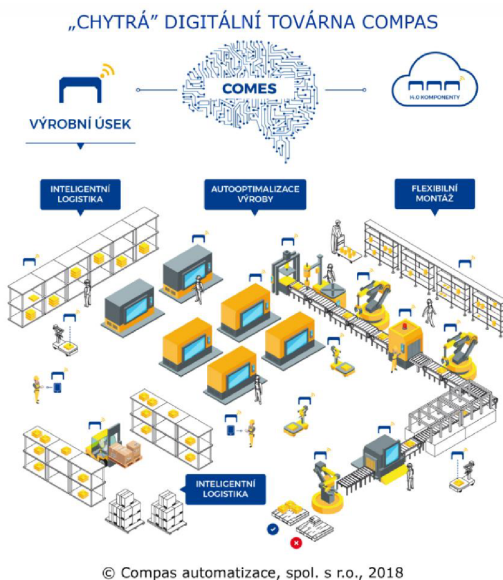
Obr. 1. 14 Koncept chytré továrny
