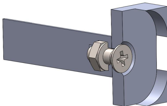
Obr. 5-2 Spojení dílu k uchycení kostky s hřídelí
