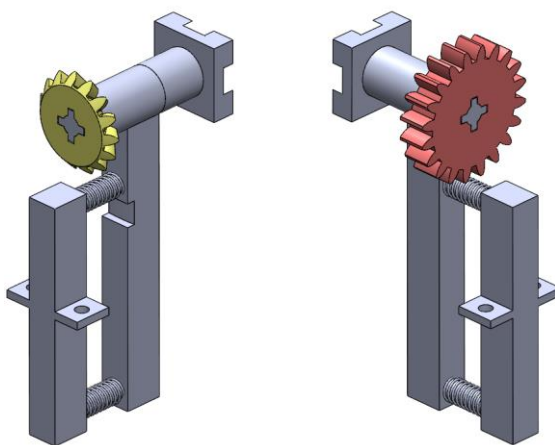
Obr. 5-9 Vedení ramen řešiče
