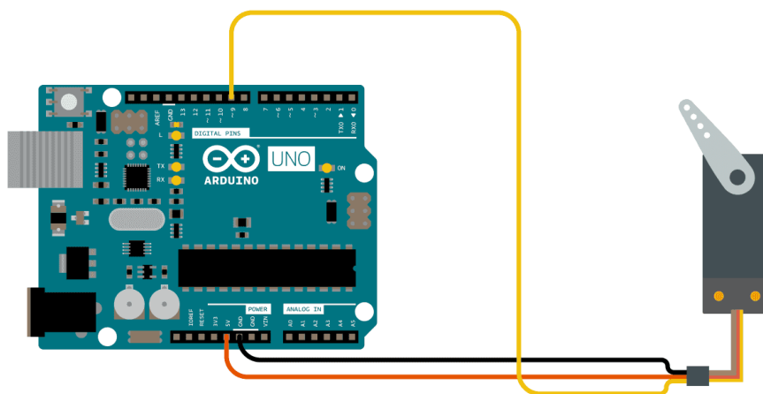
Obr. 5-13 Schéma zapojení servomotoru [22]
