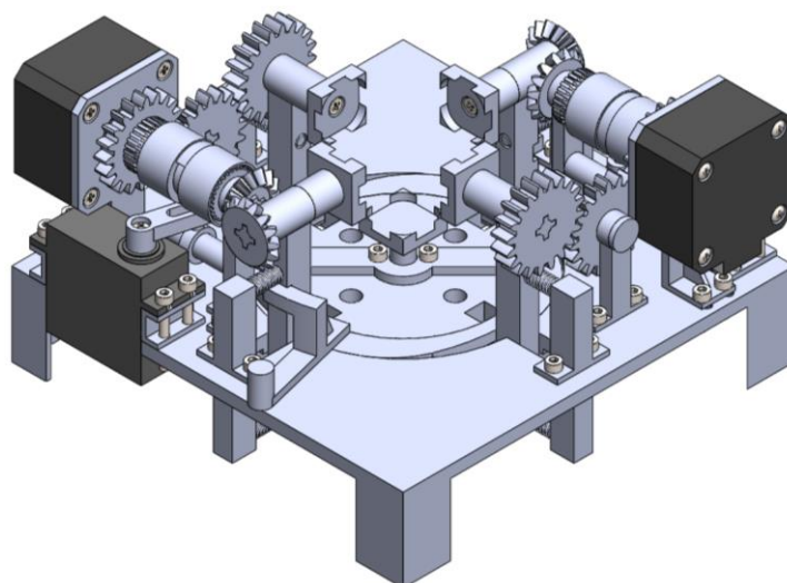
Obr. 5-12 Model řešiče Rubikovy kostky
