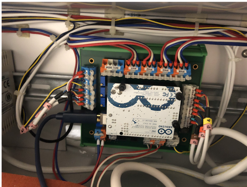
Obrázek 3.10: Řídicí jednotka GOLEM 2 – snímek ukazuje umístění a zapojení řídicí jednotky spolu se zabudovaným Arduino Uno [24]
