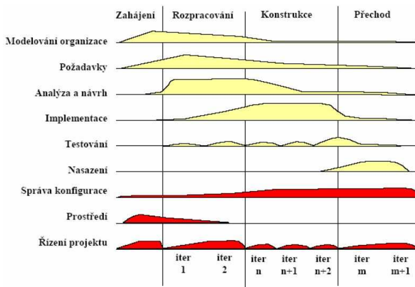
Obr. 1: Dvojdímenzionální znázornění RUP (převzato z [Lit4])
