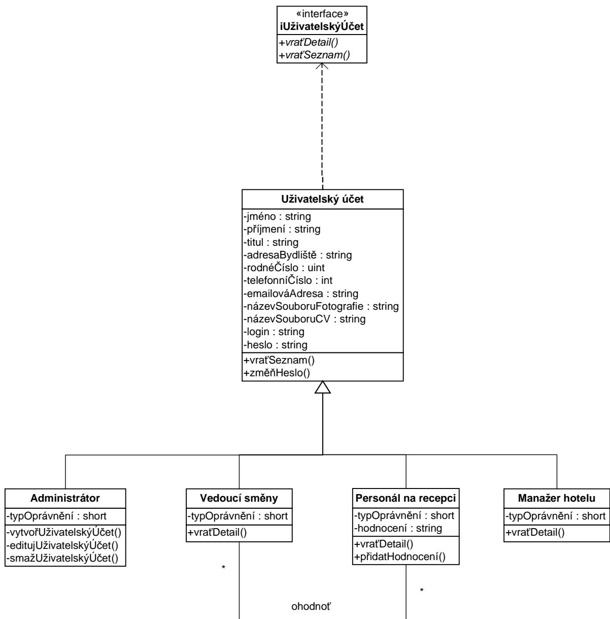
Obr. 21: Balíček Uživatelský účet
