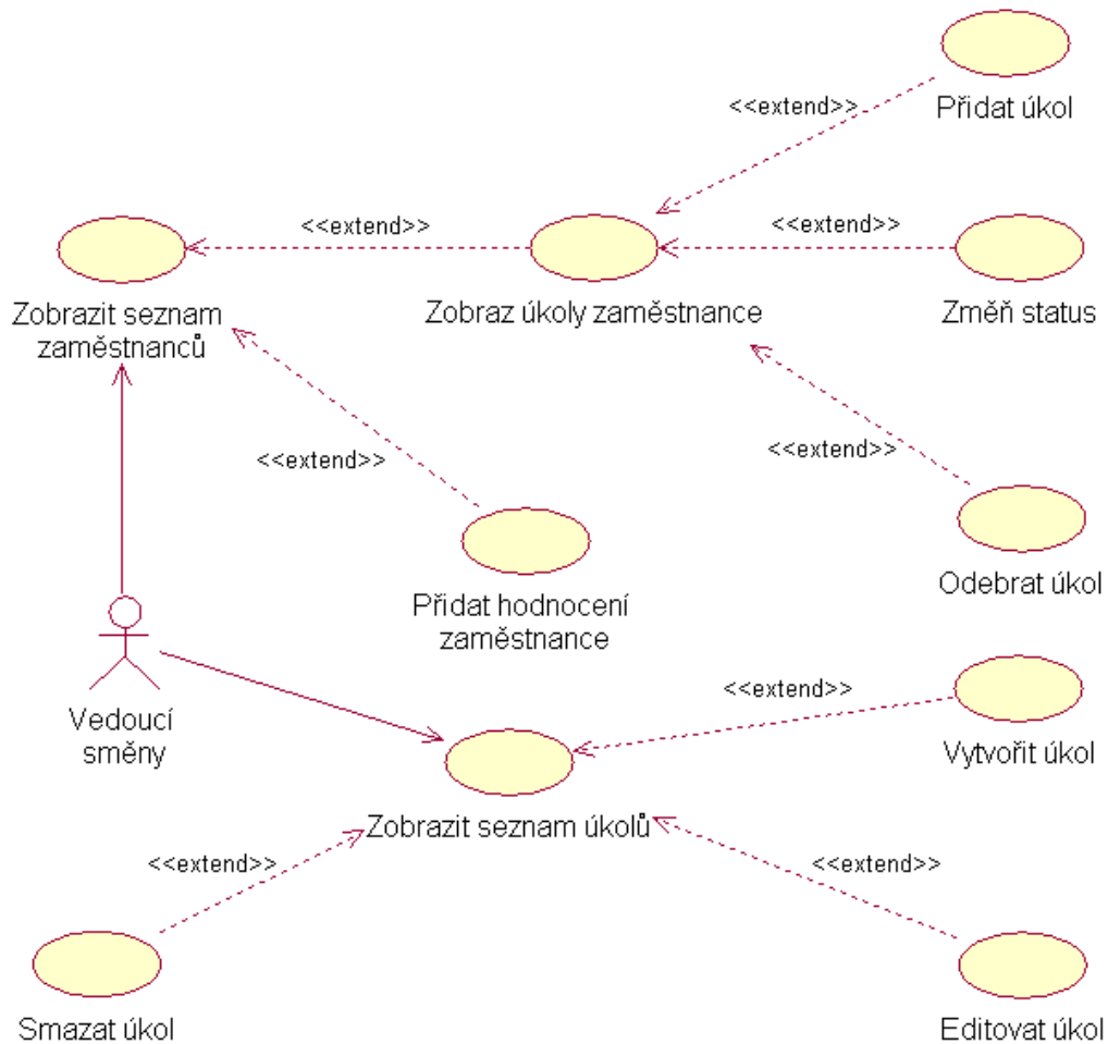
Obr. 9: Diagram případů užití
